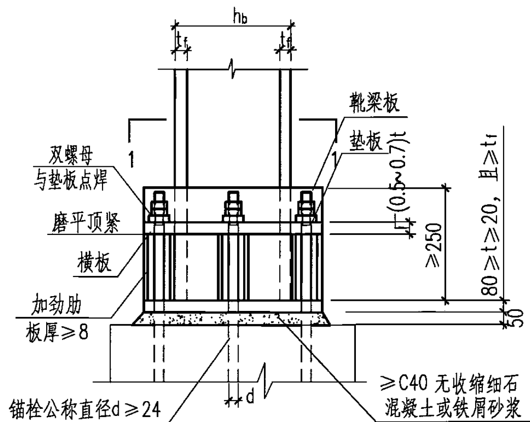
槽型靴梁的板式柱脚 (柱脚c)
