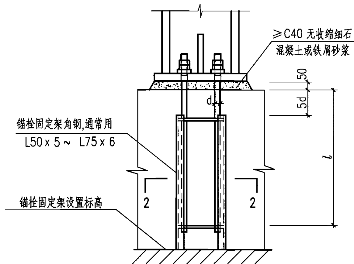
柱脚锚栓固定支架(二)
