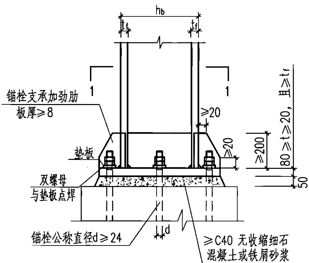
无靴梁板式柱脚(二)
