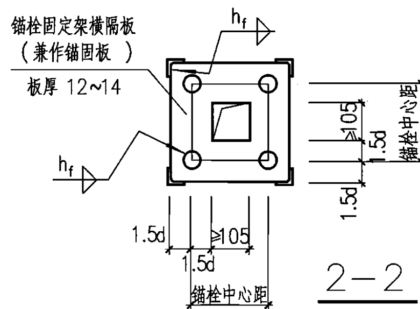
柱脚锚栓固定支架(二)
