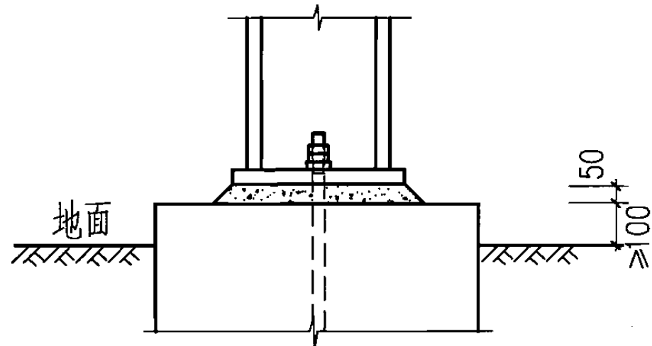
外露式柱脚在地面以上时的防护措施
