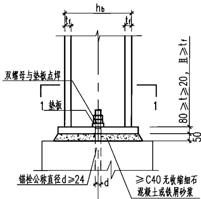
外露式铰接柱脚构造(一) (用于柱截面较小时)
