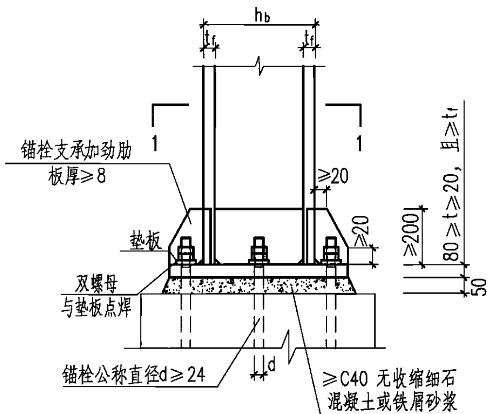
无靴梁板式柱脚(一) (柱脚a)
