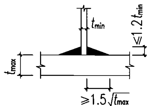
图7.2 不等焊脚尺寸角焊缝
