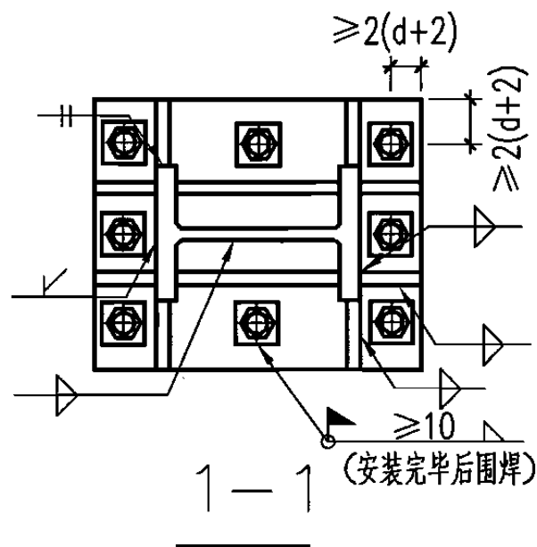
无靴梁板式柱脚(一) (柱脚a)
