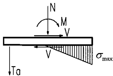
图4.2.2 计算简图
