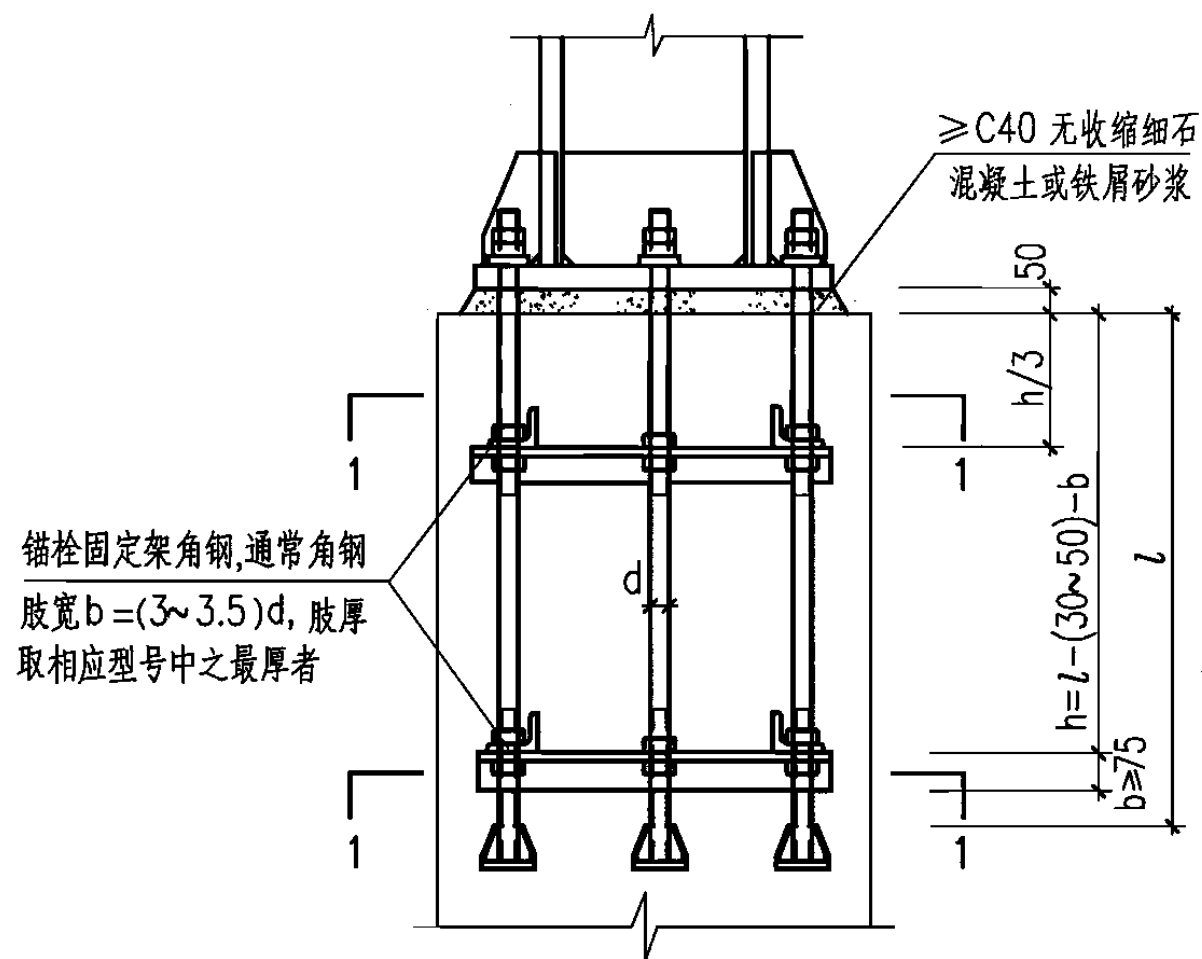
柱脚锚栓固定支架(一)
