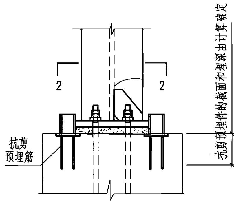
外露式柱脚抗剪键的设置(二)
