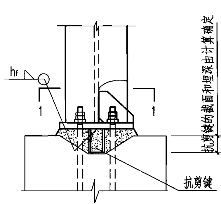
外露式柱脚抗剪键的设置(一)
