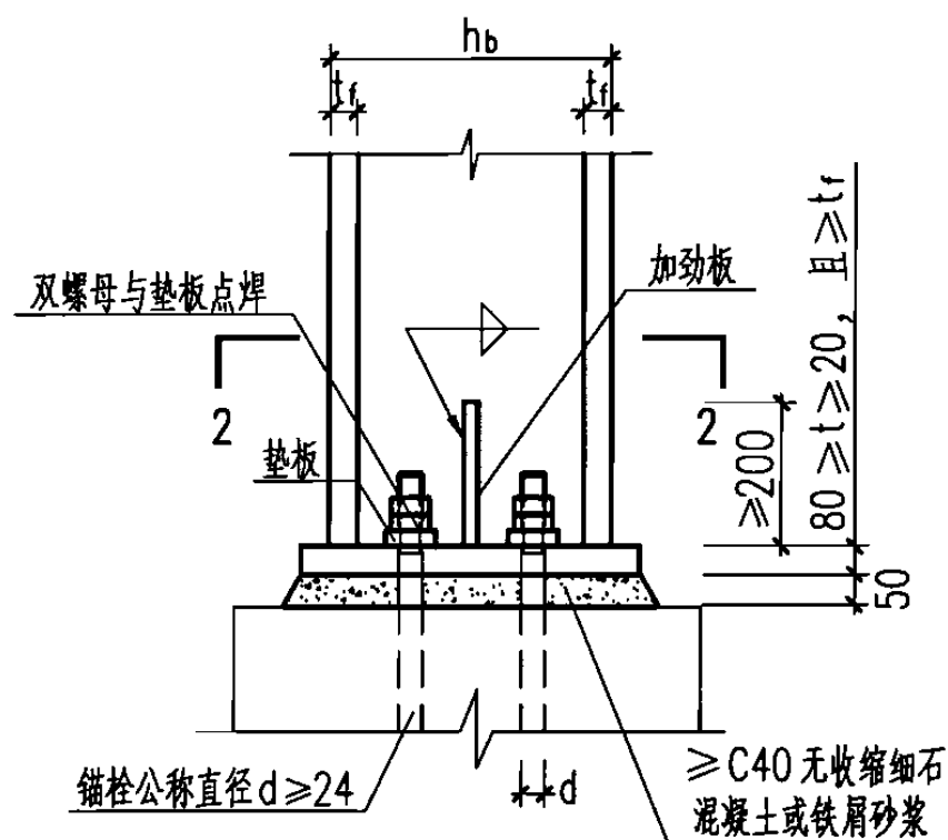
外露式铰接柱脚构造(二) (用于柱截面较大时)
