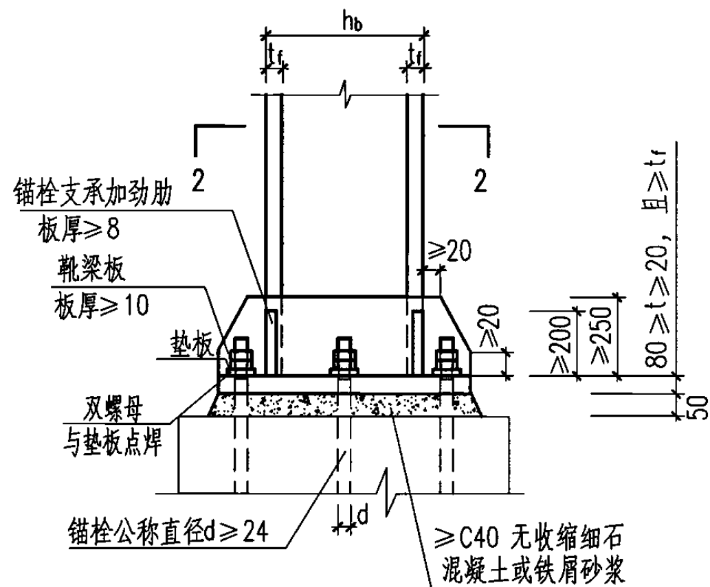
T型靴梁的板式柱脚
