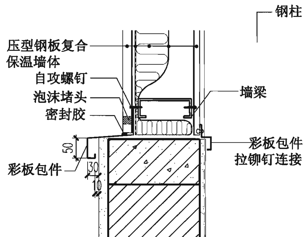
⑥ 墙脚
