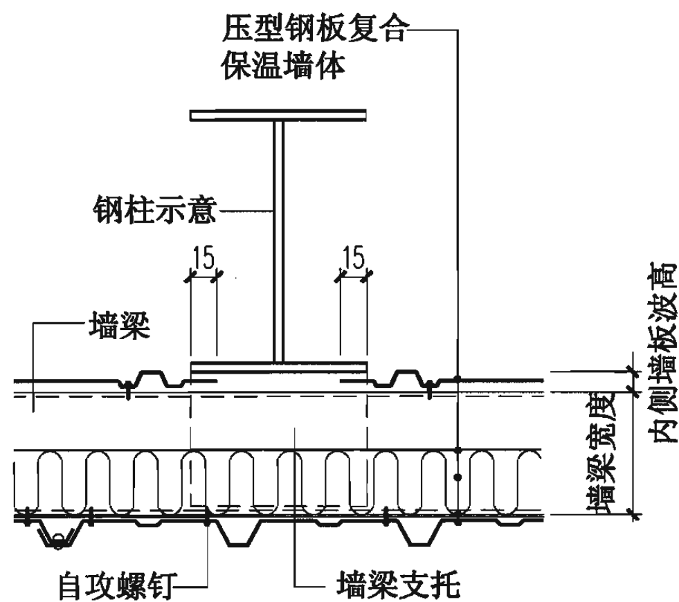
② 遇柱处
