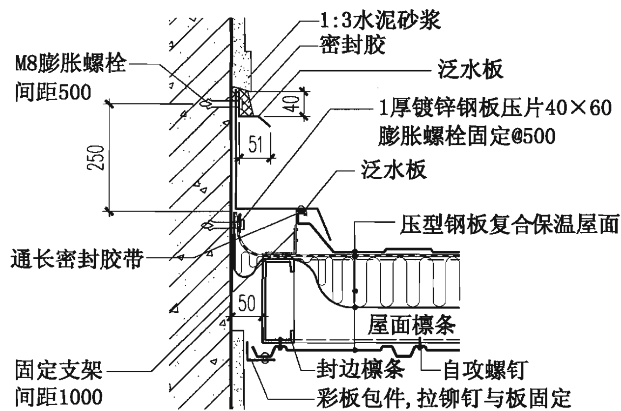
19 高低跨
