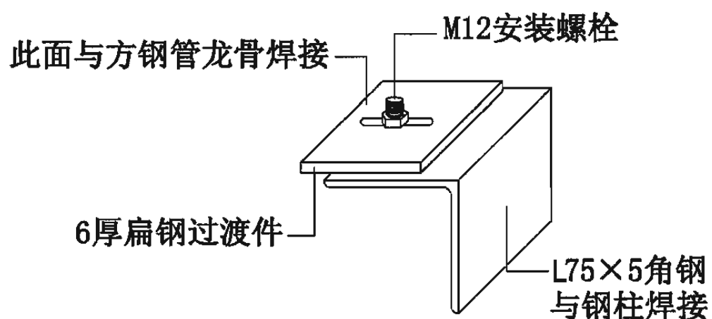
方钢管龙骨端部连接大样图
