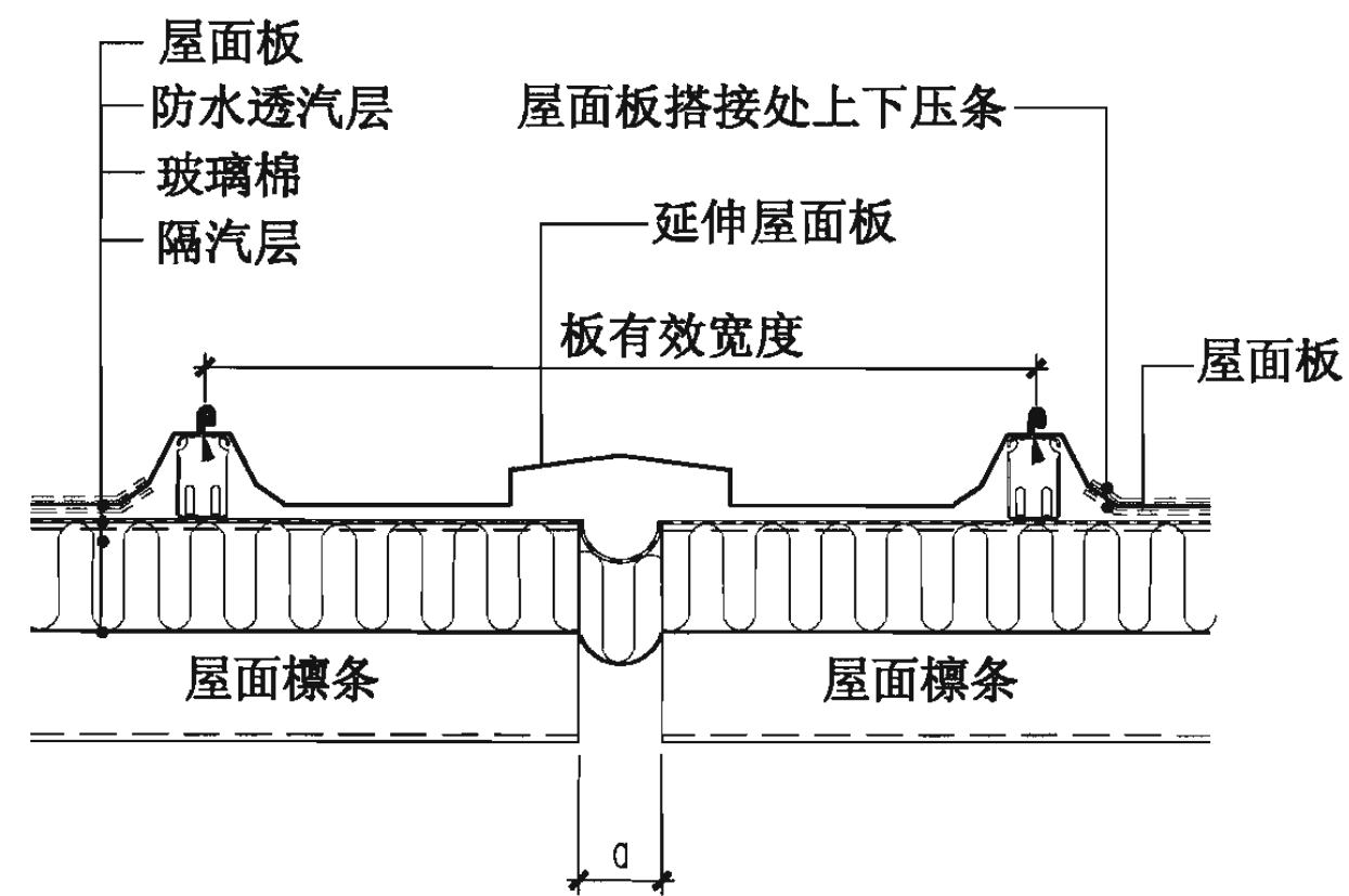
9 变形缝
