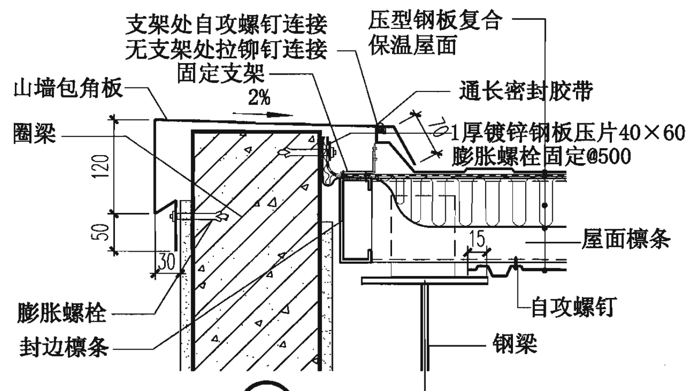
16 单坡屋脊
