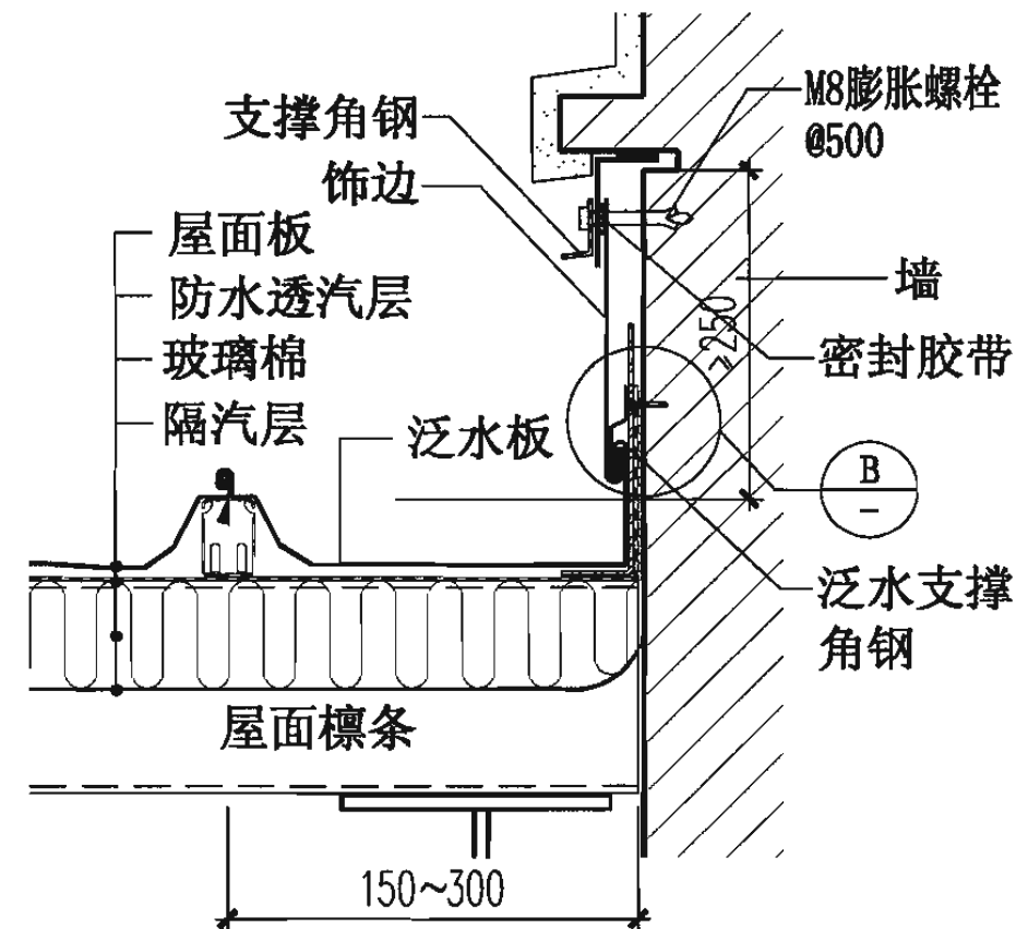
⑪ 高低跨
