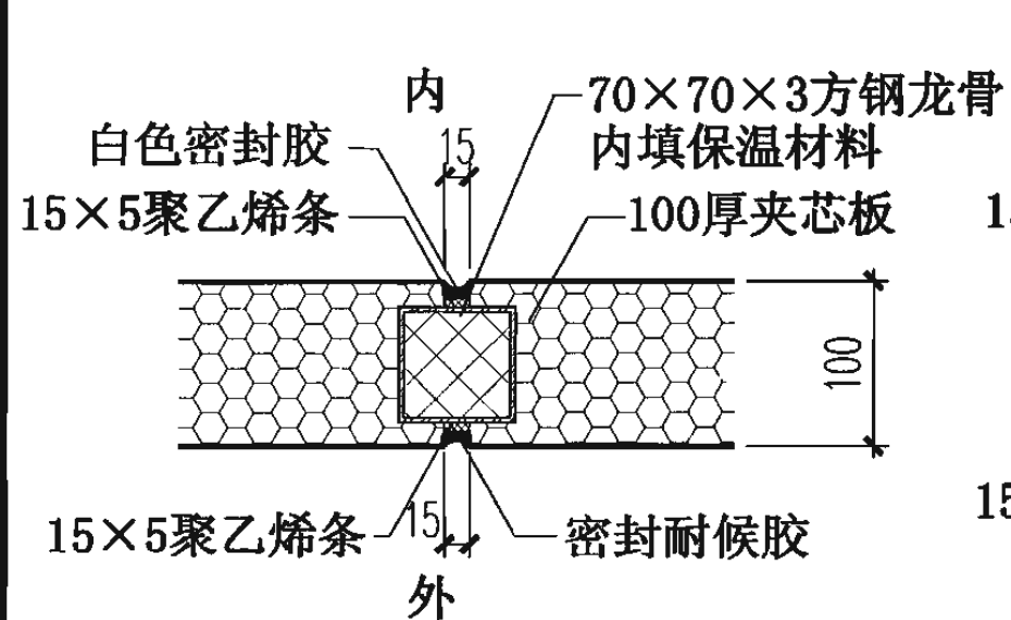
100厚墙板拼接
