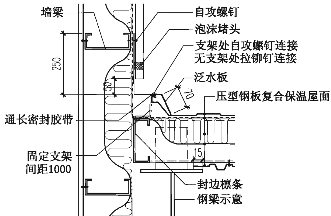
21 高低跨
