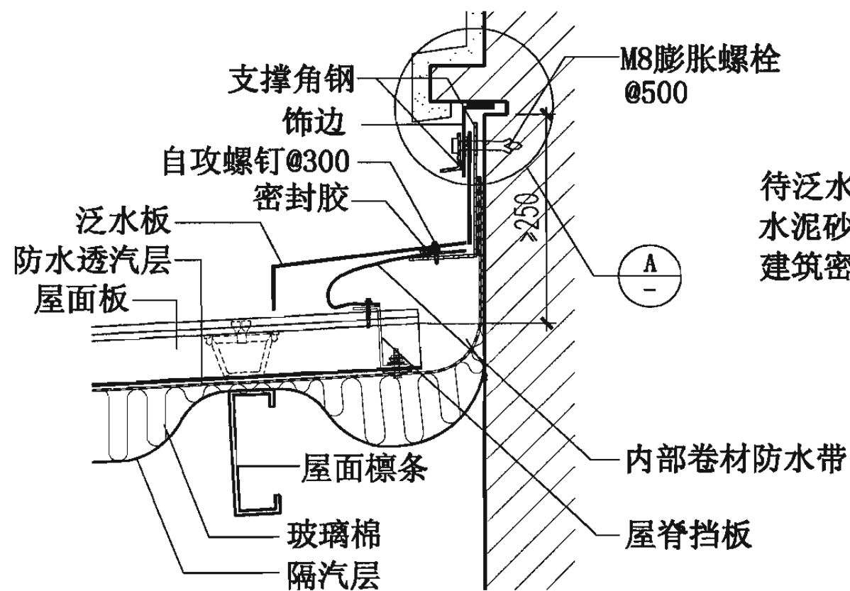
⑩ 高低跨
