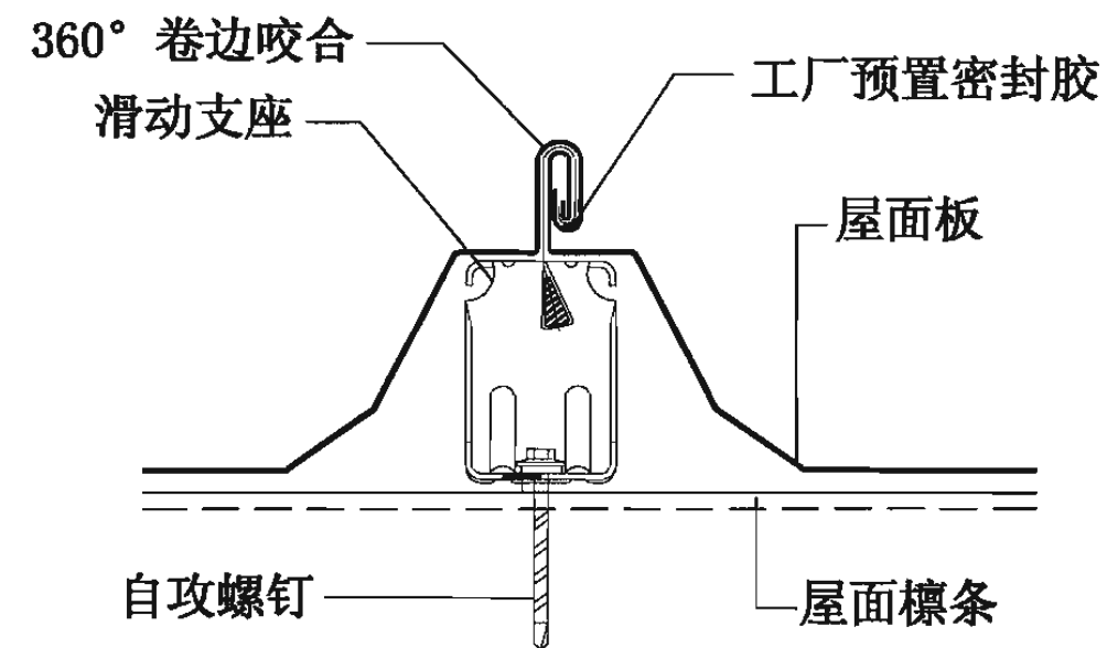
锁边示意
