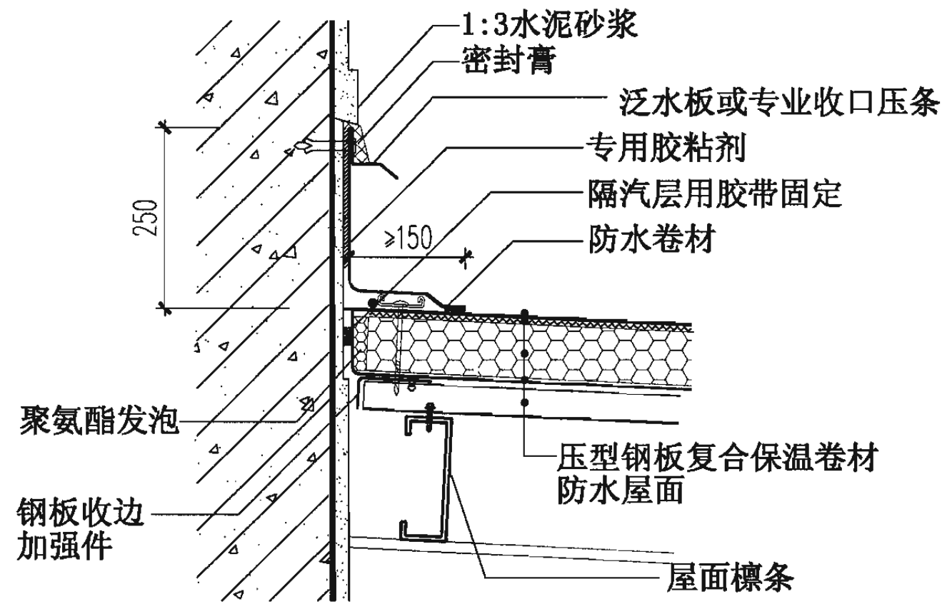
⑩ 高低跨
