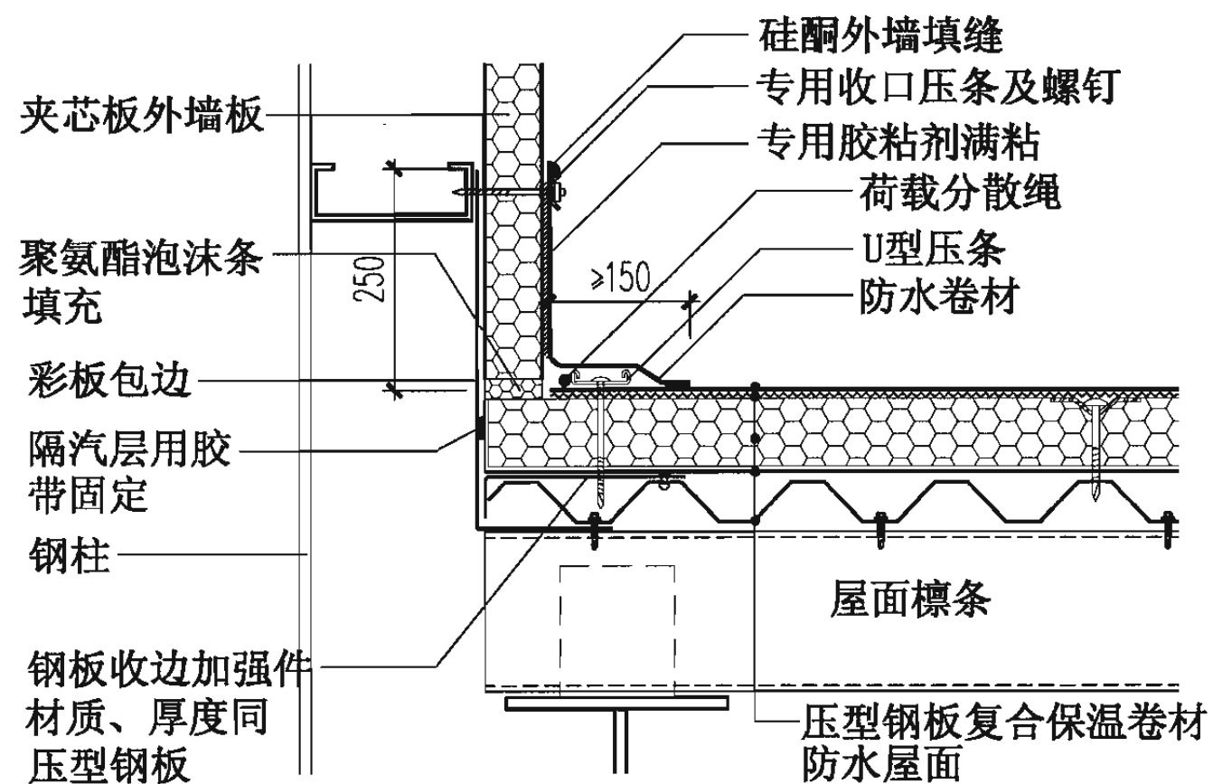
⑪ 高低跨
