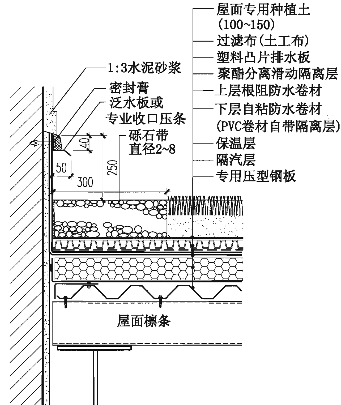
女儿墙
