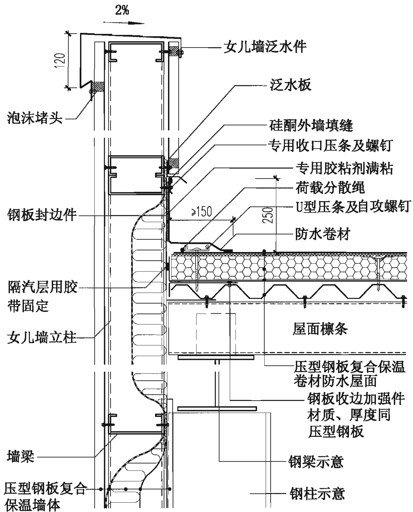
15 女儿墙
