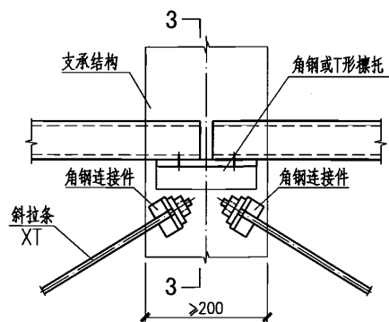
6 斜拉条与角钢连接构造
