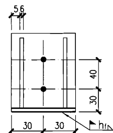
双层斜拉条角钢
