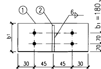
CT3 T形檩托
