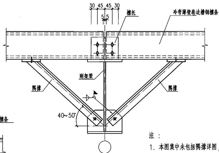
双层板隅撑安装节点
