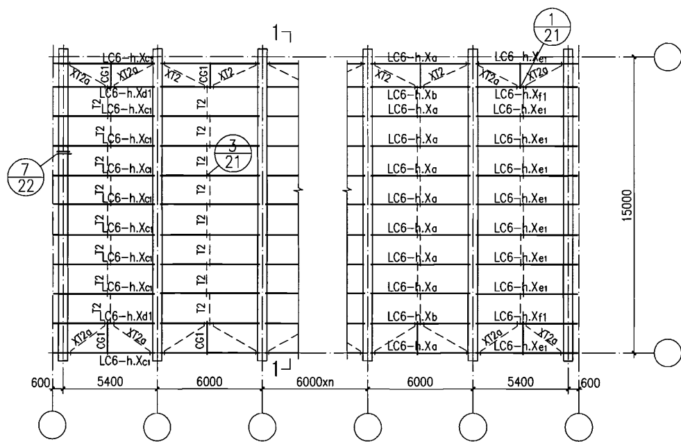
標条布置示例图（六）
