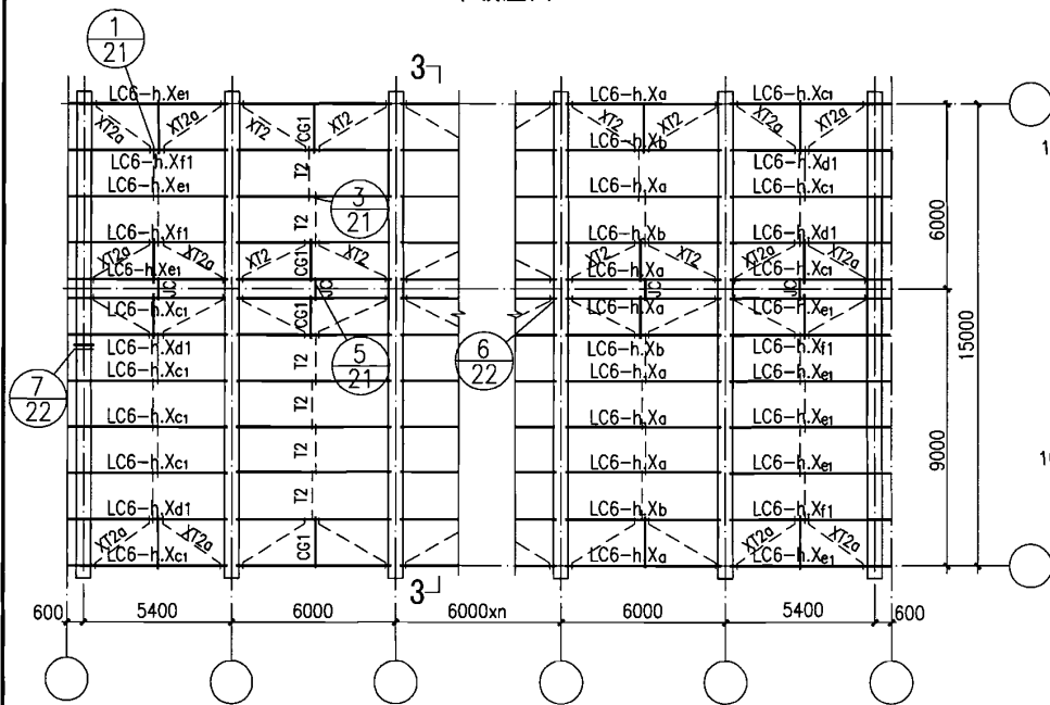
標条布置示例图 (八)
