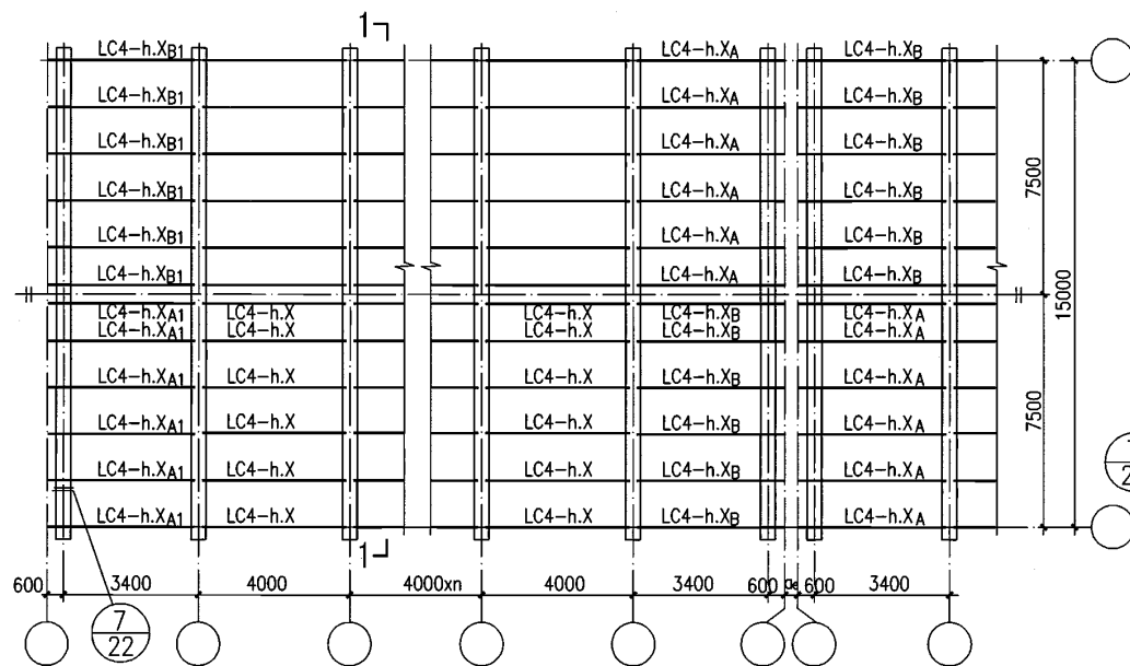
檩条布置示例图 (一)
