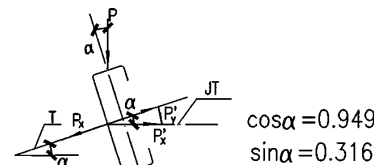
图4 脊檩受力图
