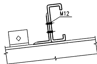
3-3 (角钢檩托)
