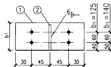
CT3 T形檩托
