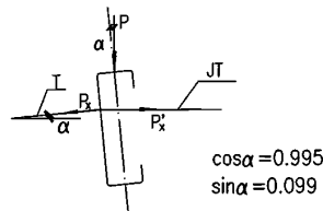
图2 脊檩受力图
