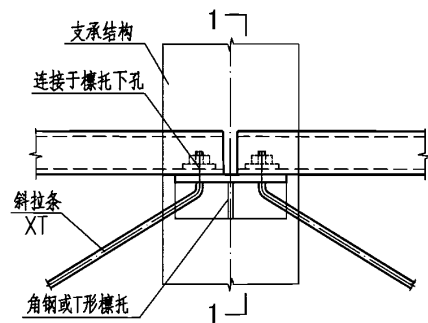
6 斜拉条与檩托连接构造
