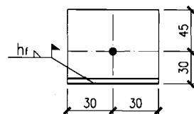
单层斜拉条角钢
