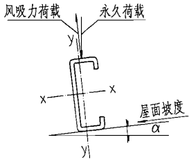
檩条线荷载作用方向与槽口朝向示意图
