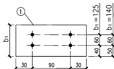
CT4 单板檩托
