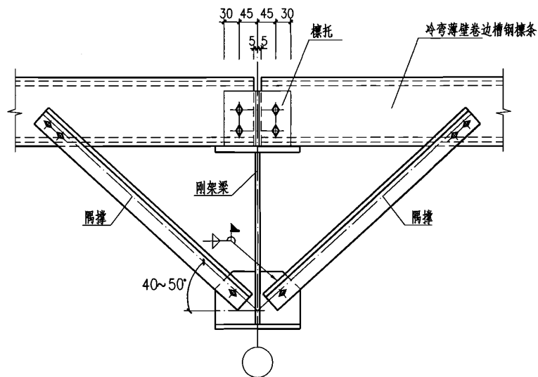
单层板隅撑安装节点
