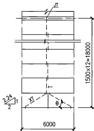
图1 檩条的拉条平面布置图
