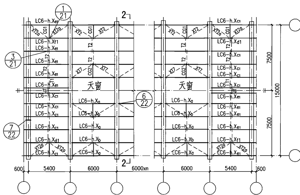
標条布置示例图（七）
