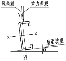
檩条线荷载作用方向与槽口朝向示意图
