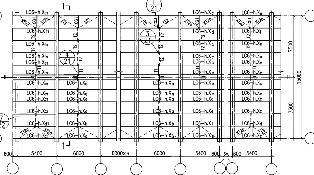
檩条布置示例图 (二)
