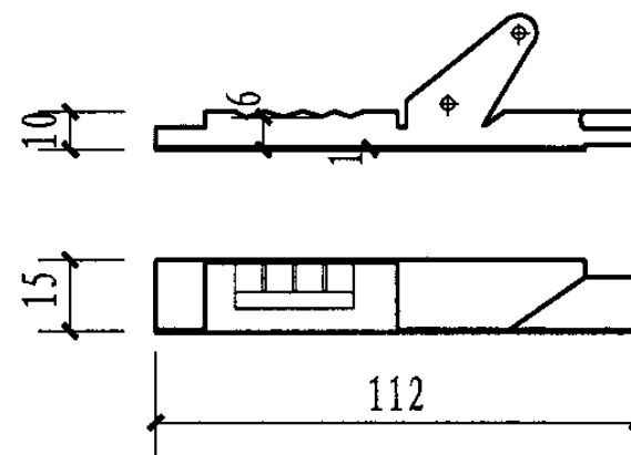
不锈钢卡夹
