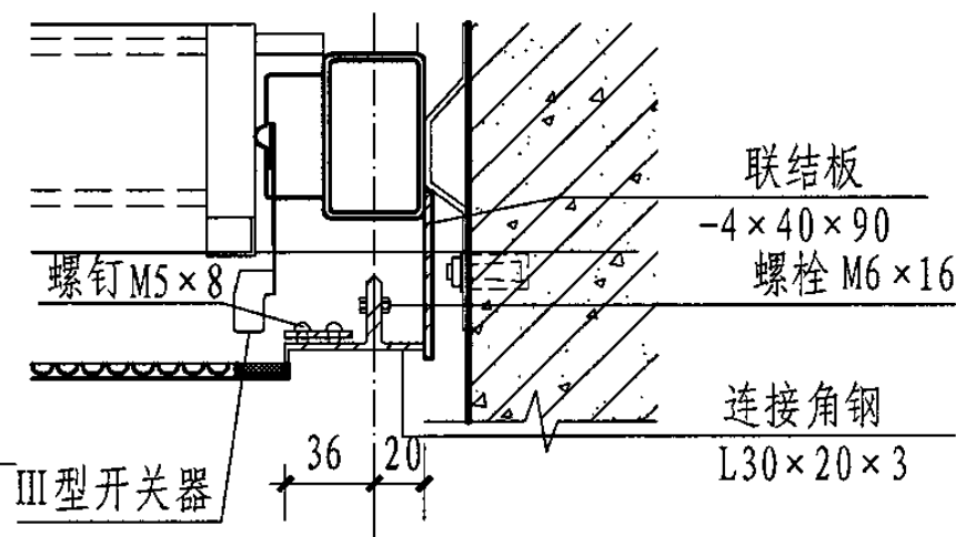
活动钢、不锈钢百叶窗纱窗安装节点
