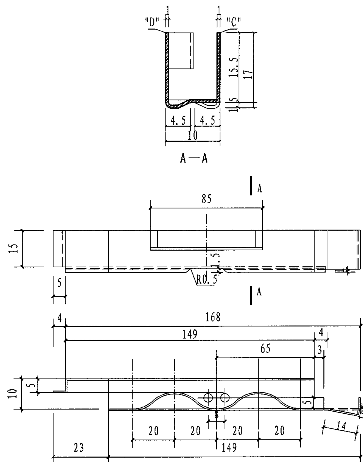
右固定夹
