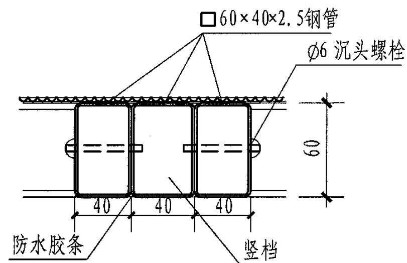
6 拼槓连接
