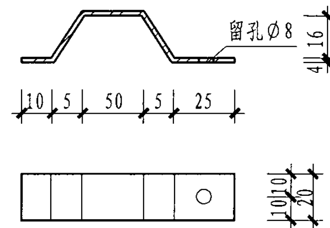
铁脚
