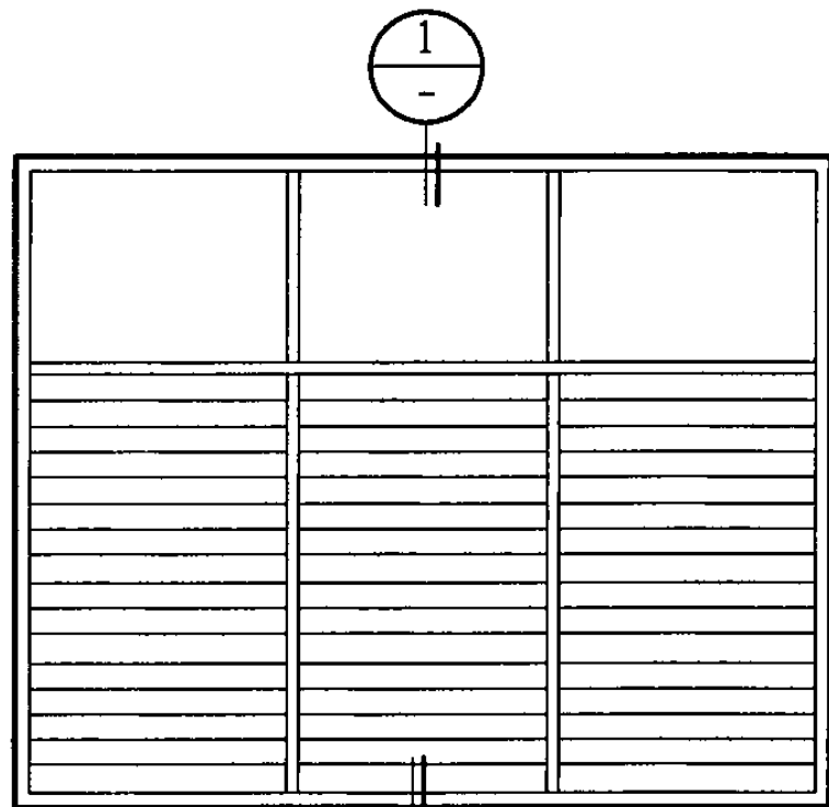
立面图一
