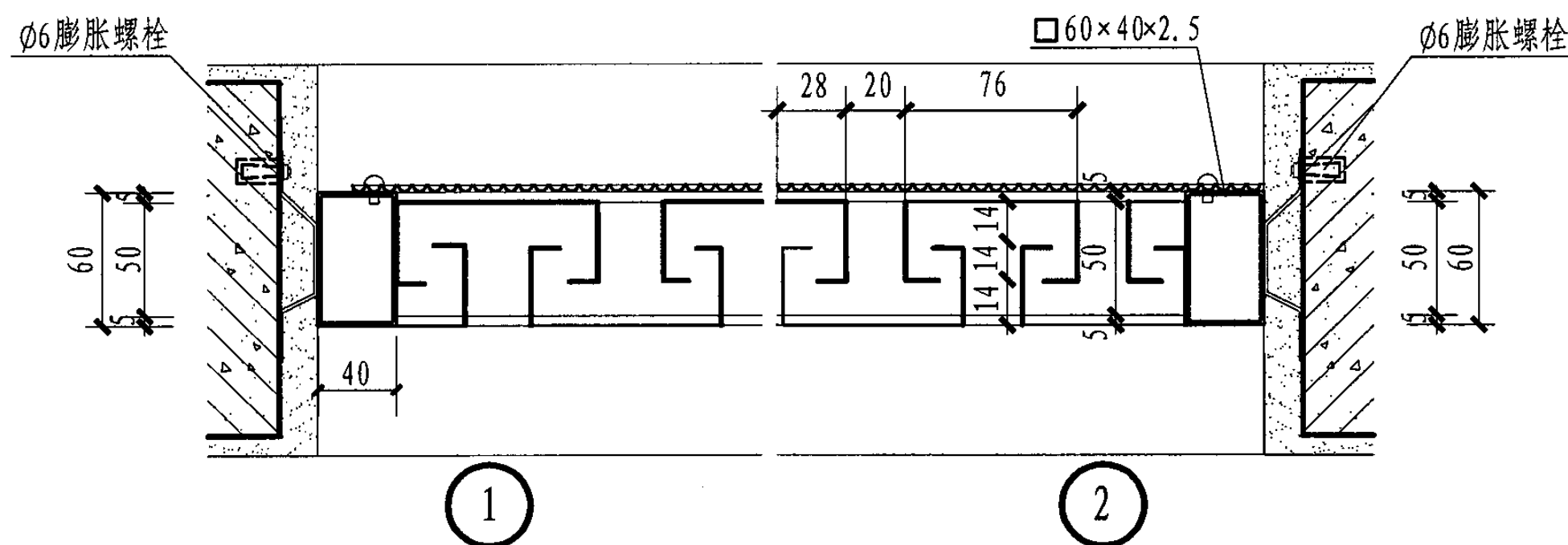
立面图
