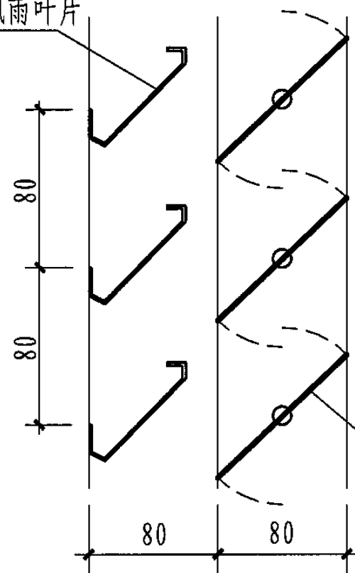
叶片形式
