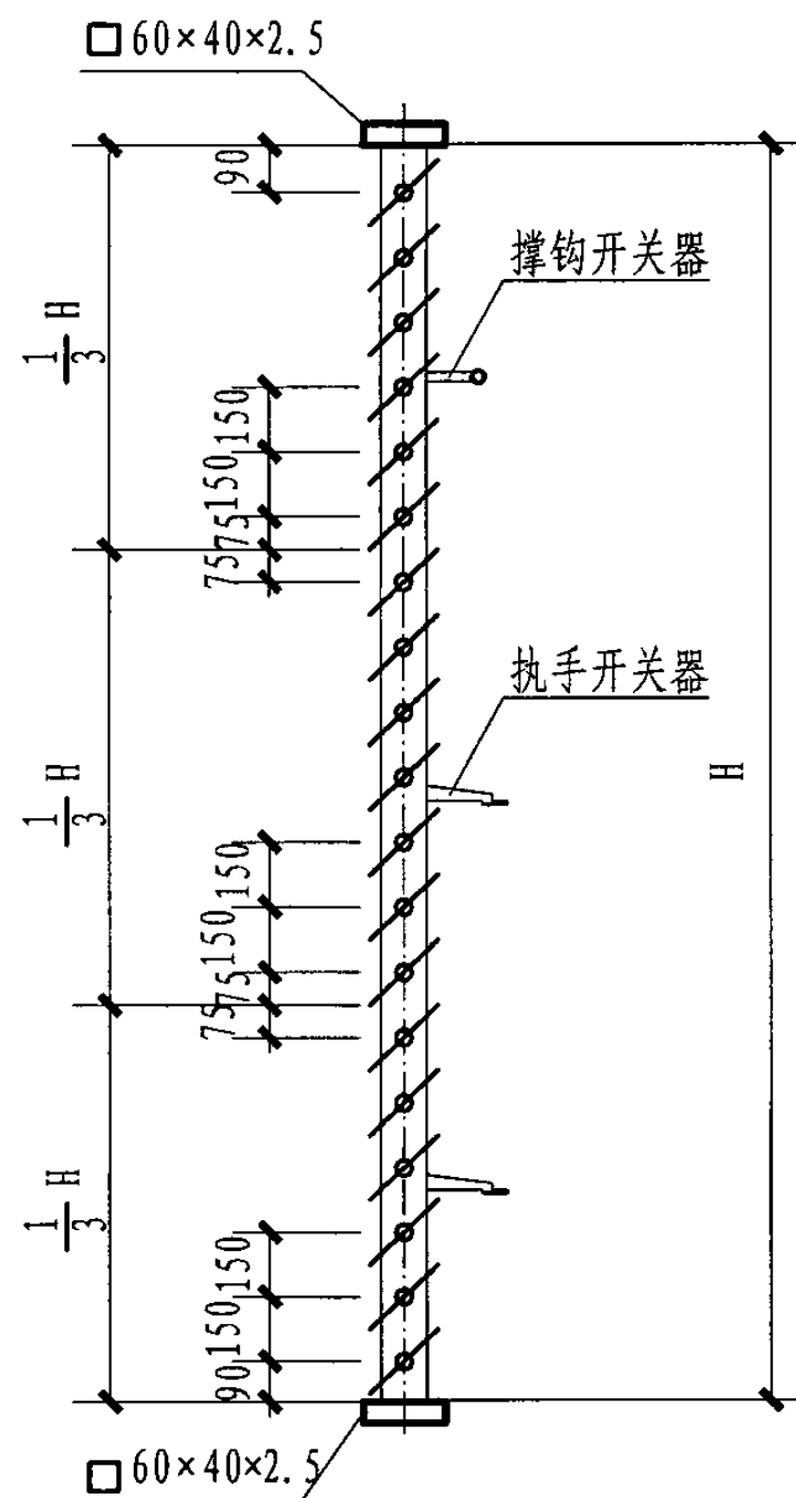
1-1剖面图
