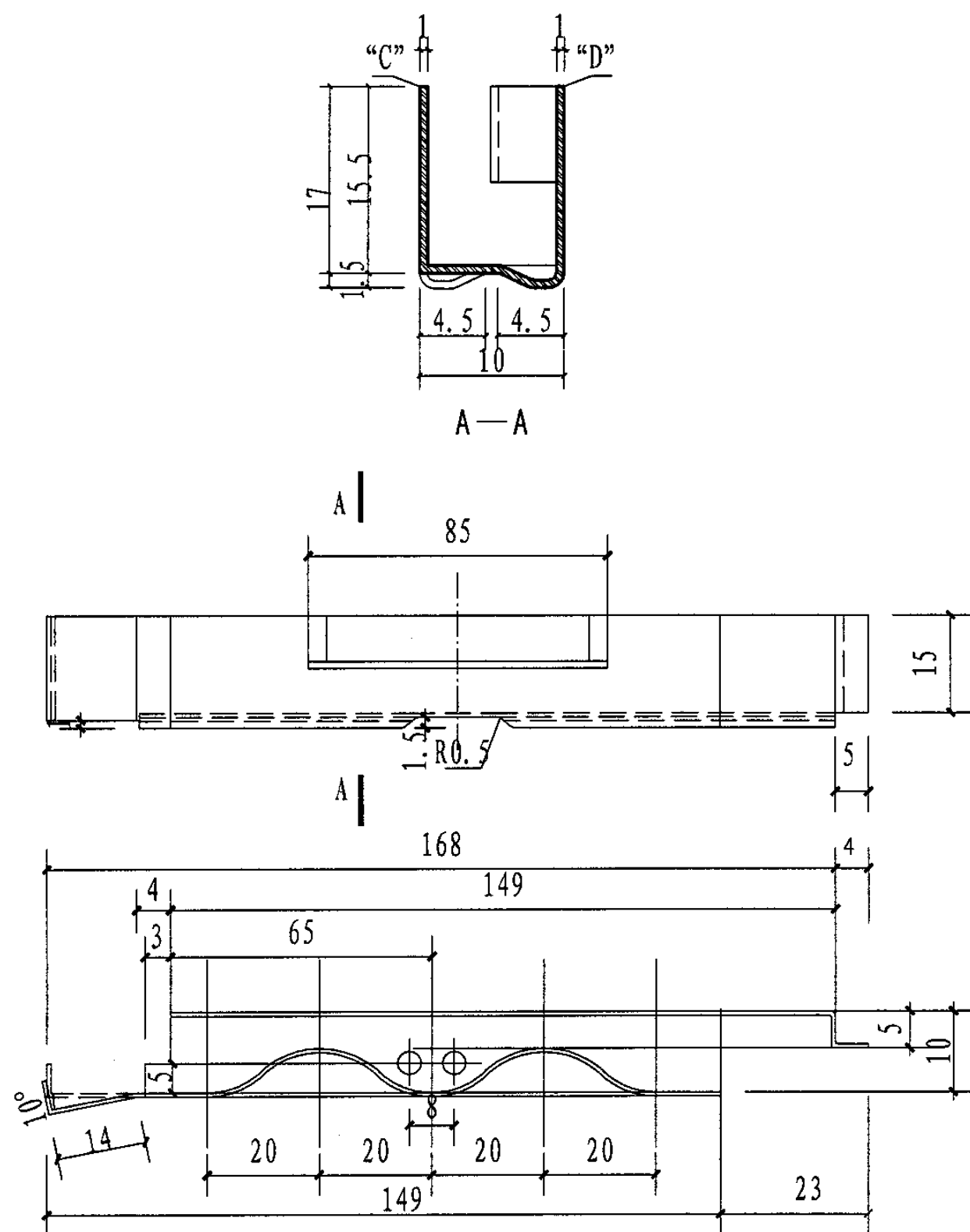
左固定夹
