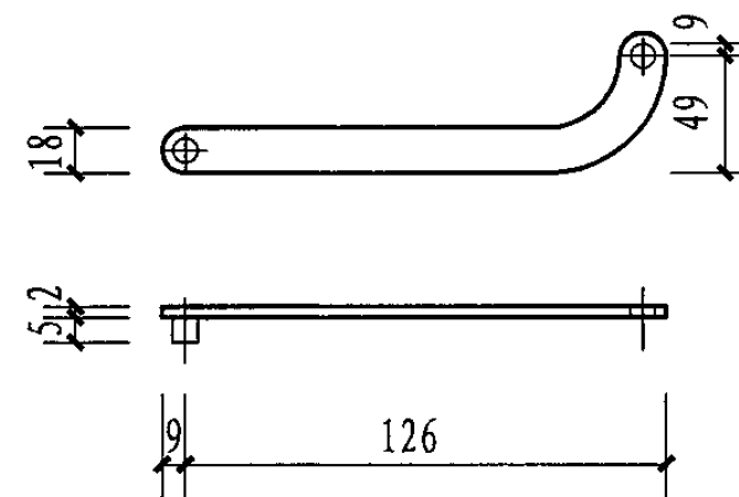
不锈钢曲臂
