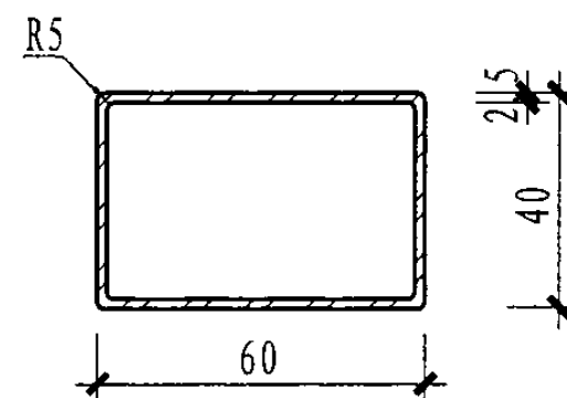
钢窗框
