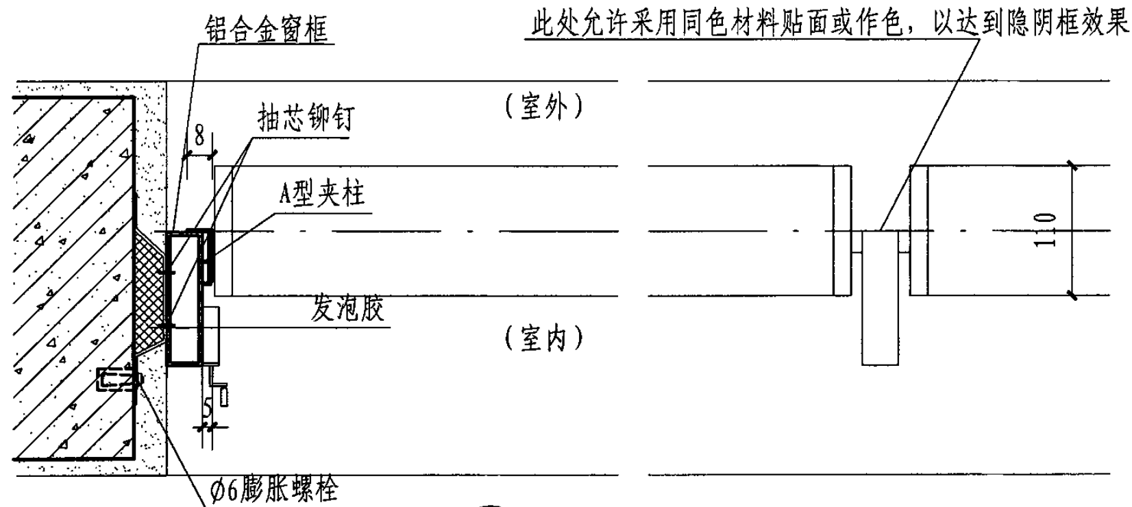
1 A型夹柱
