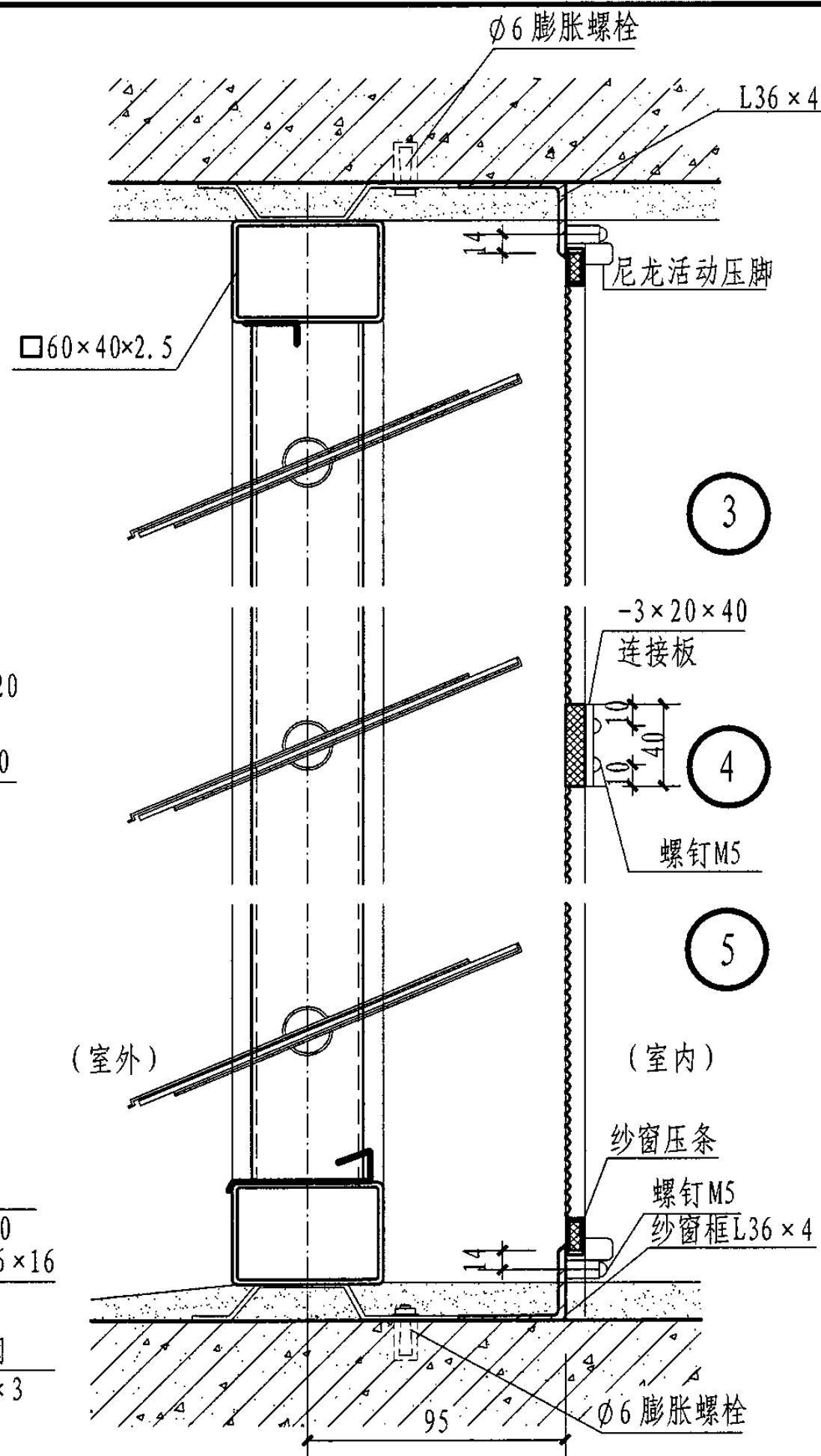
活动钢、不锈钢百叶窗纱窗安装节点
