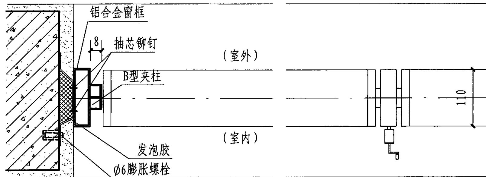
2 B型夹柱
