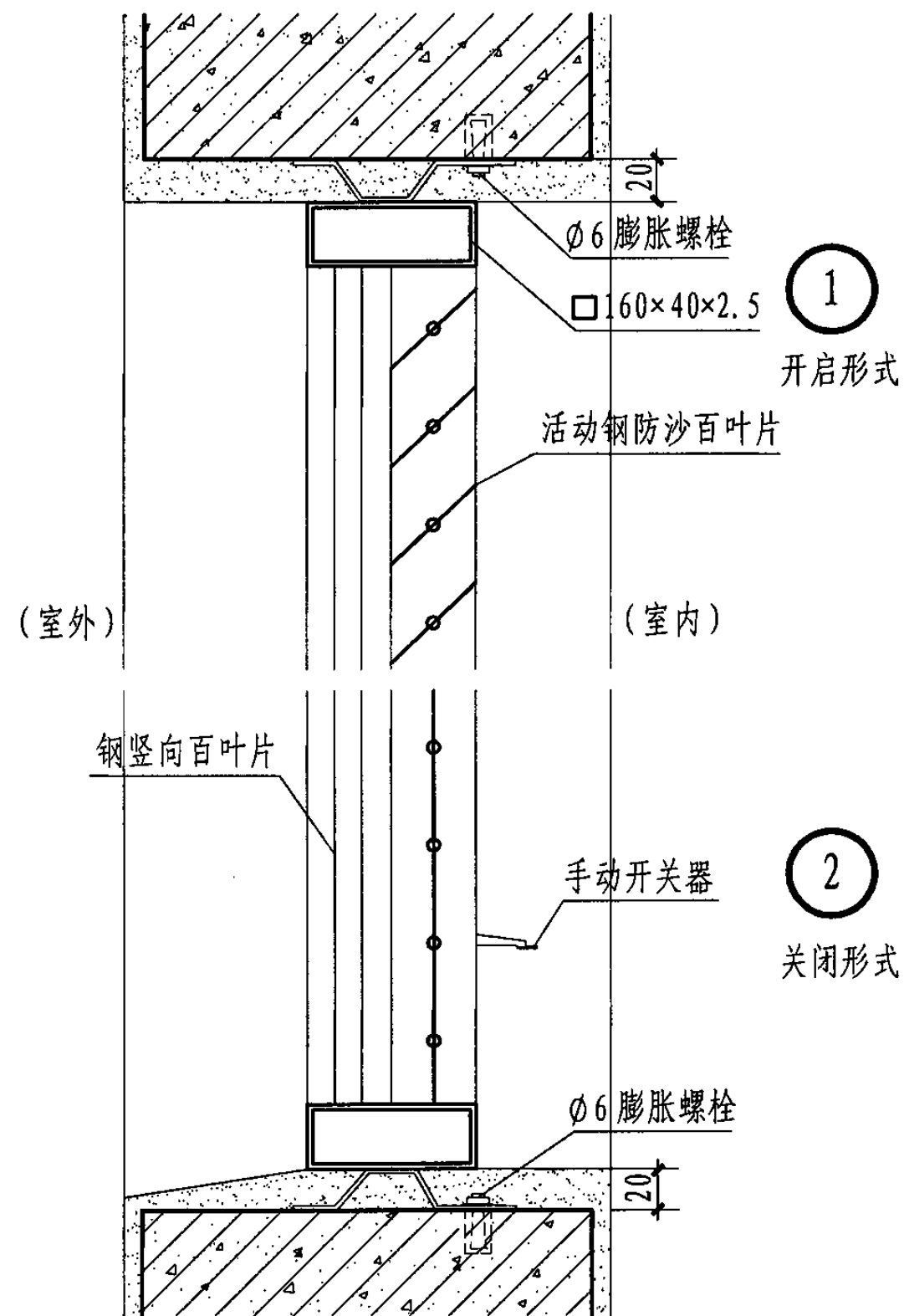
叶片形式
