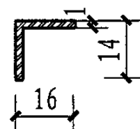
上挡水板
