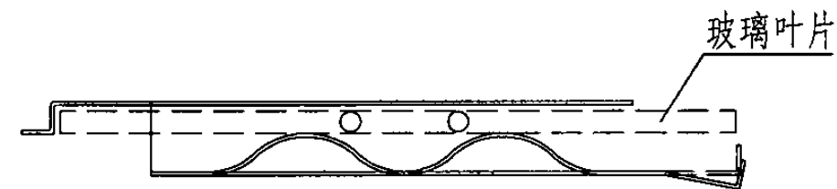
不锈钢固定夹
