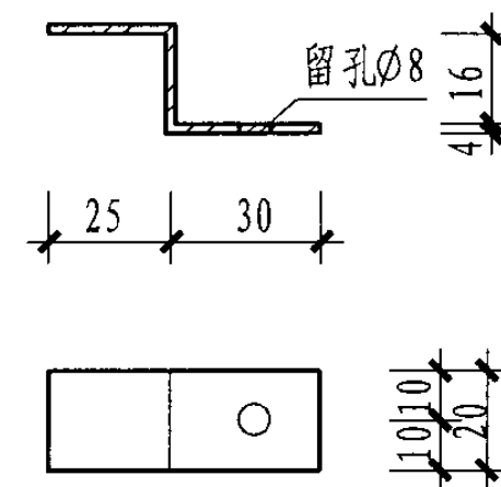
Z型铁脚
