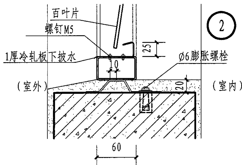
剖面图(混凝土墙)
