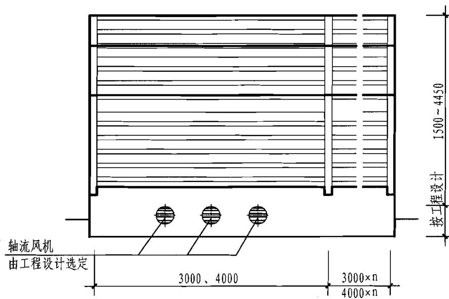
立面图
