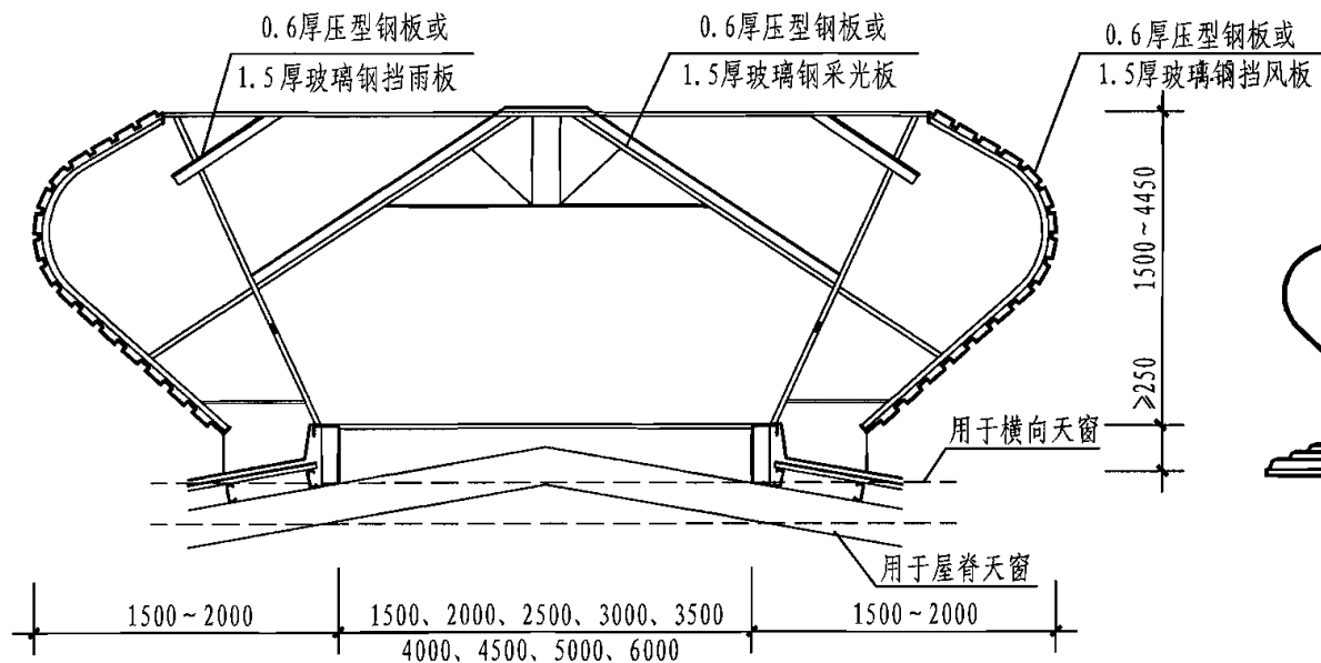
剖面图
