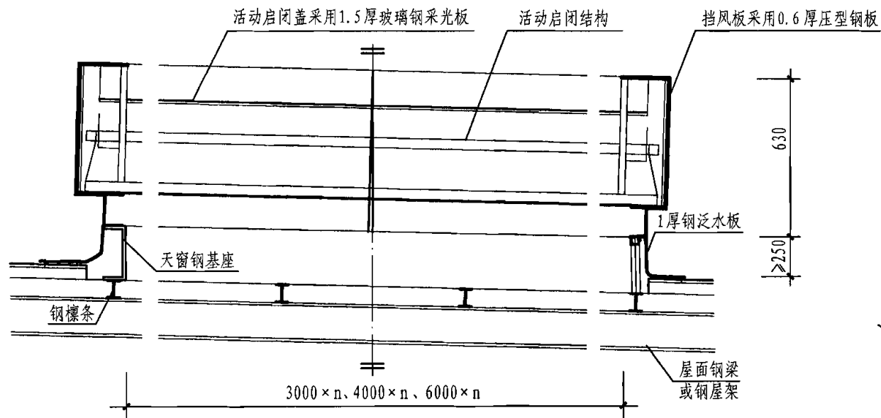
1-1 剖面图
