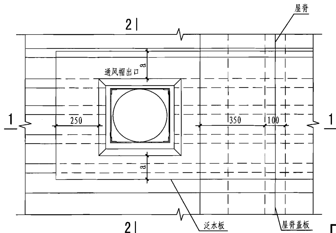
平面图
