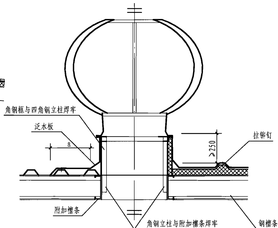
2-2 剖面图
