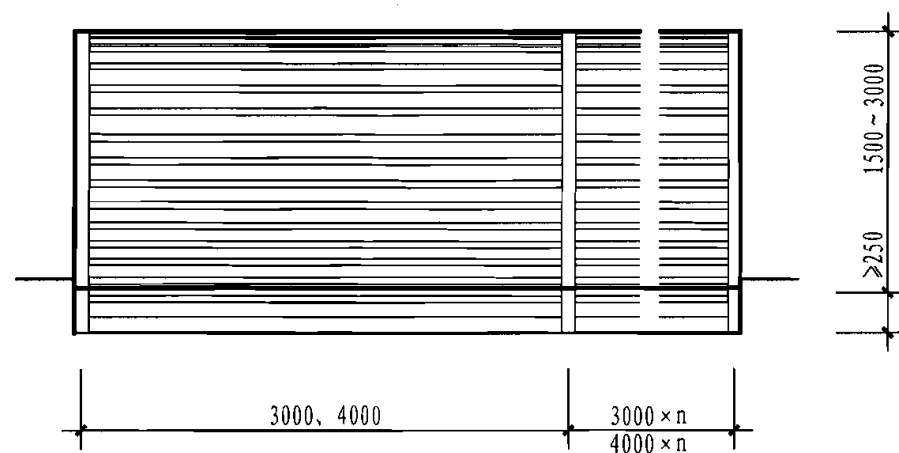
立面图
