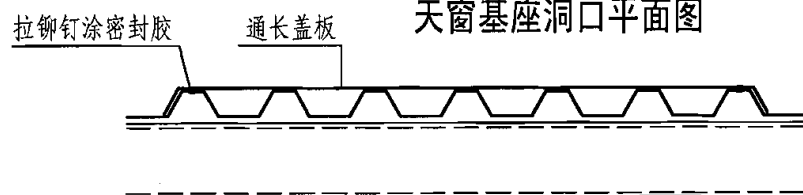
2-2 剖面图
