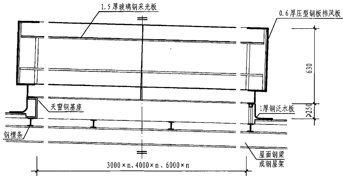
1-1 剖面图
