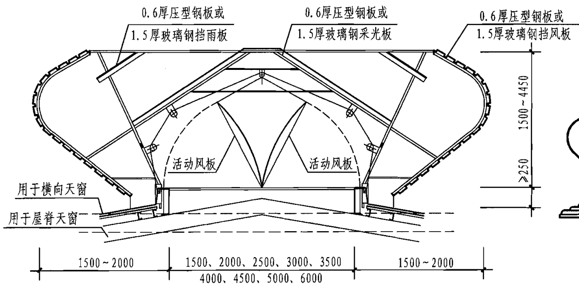
剖面图
