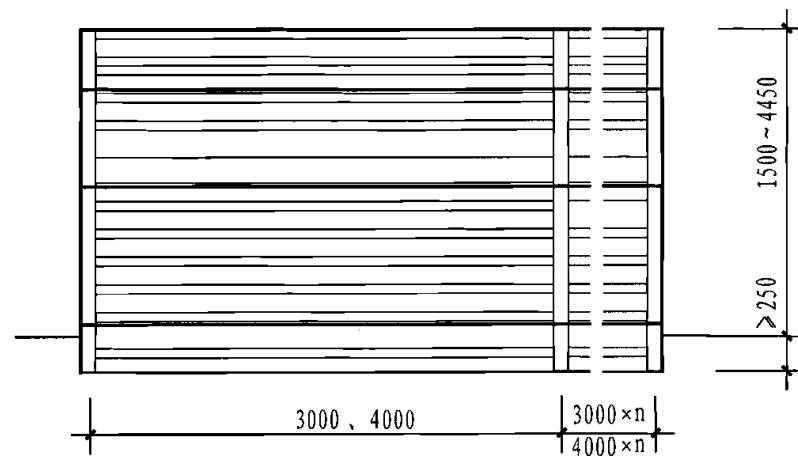
立面图
