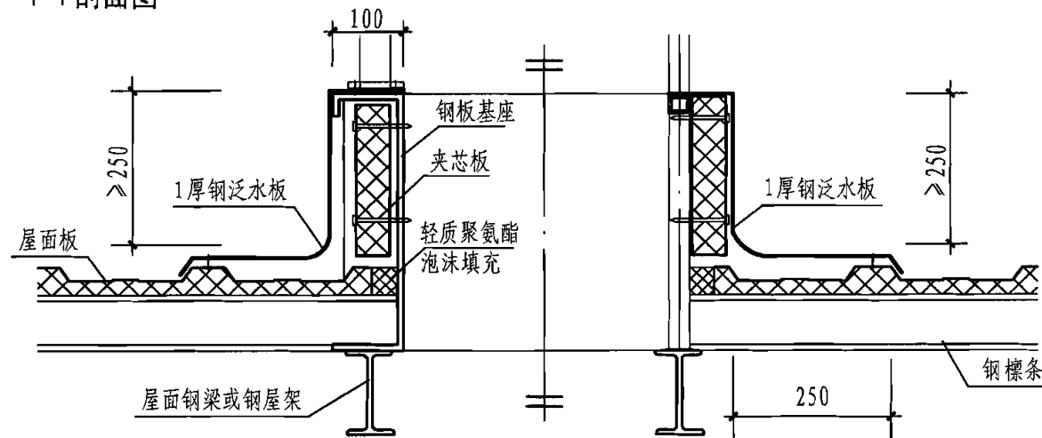
2-2 剖面图
