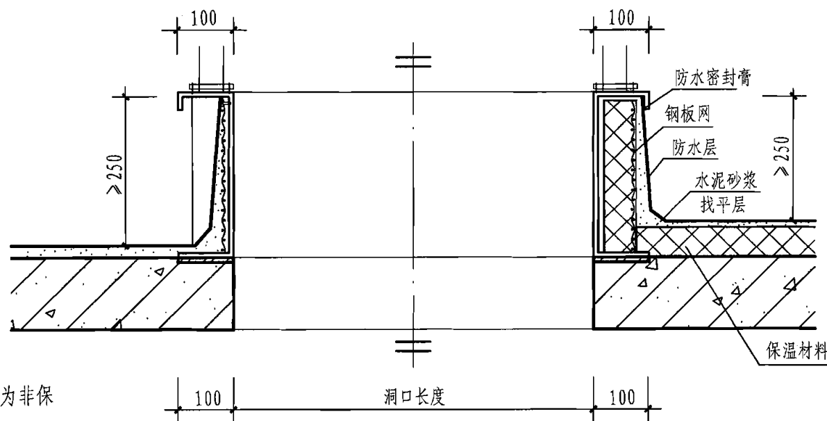
2-2 剖面图
