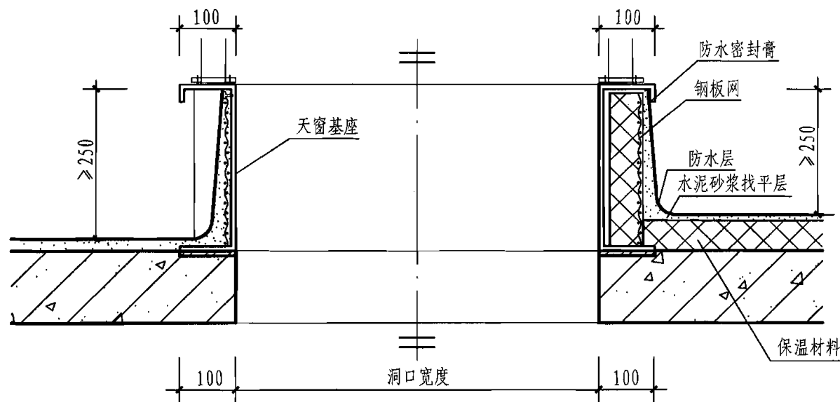
1-1 剖面图
