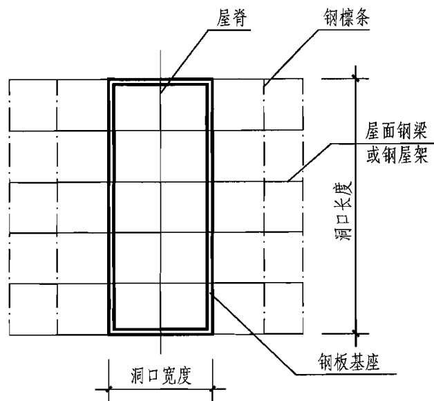
屋脊天窗平面示意图
