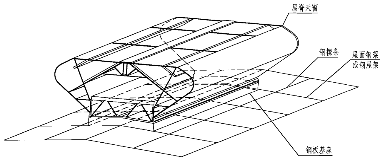
屋脊天窗示意图
