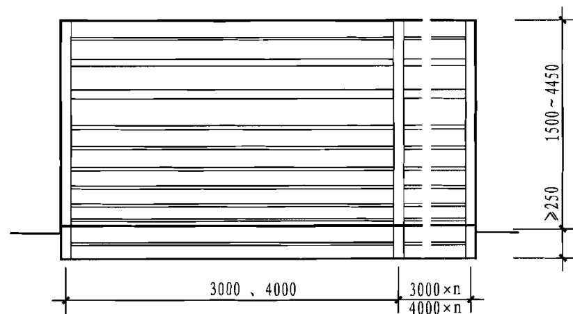
立面图
