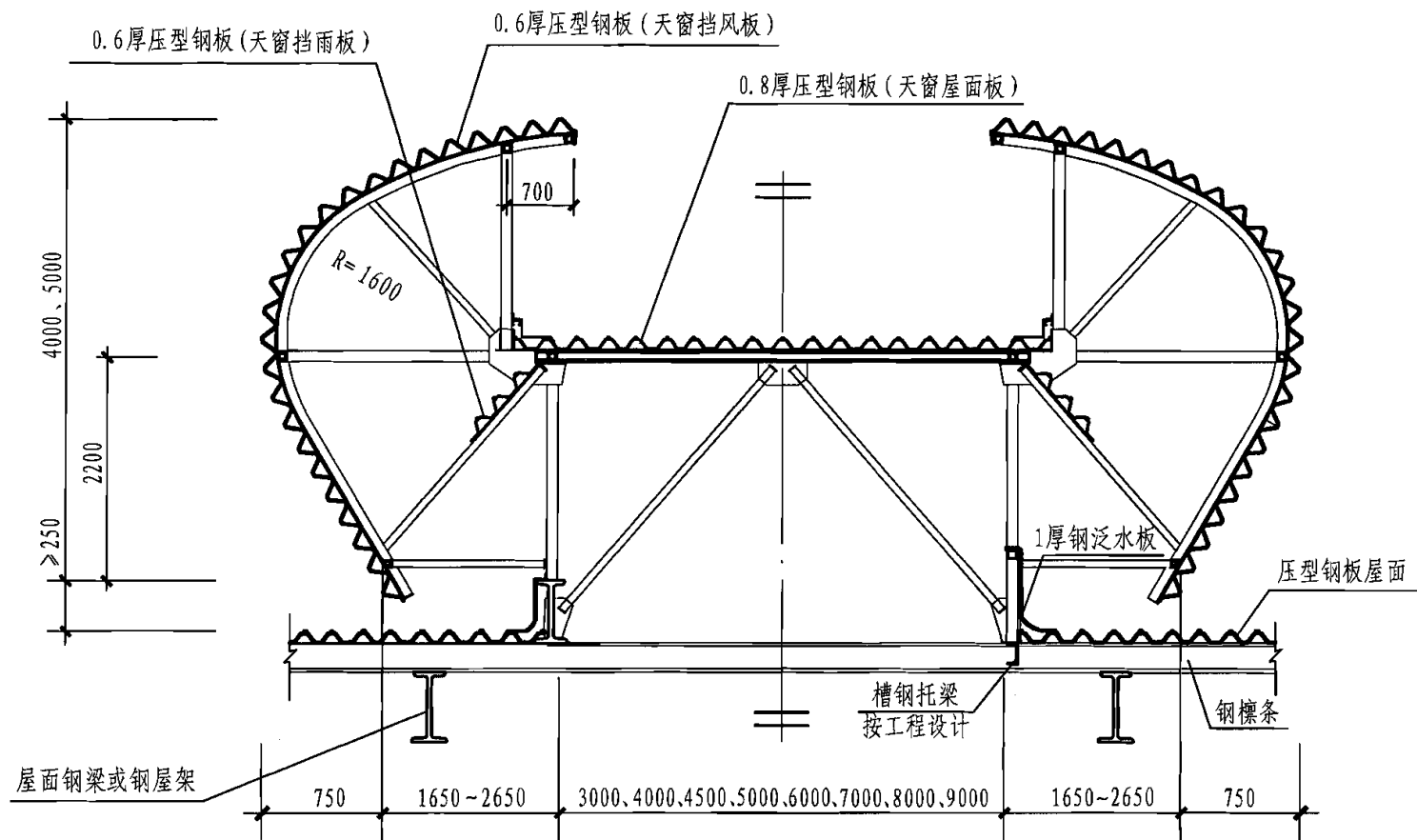
B-B 剖面图
