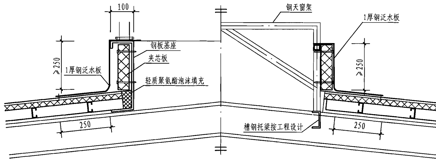
1-1 剖面图
