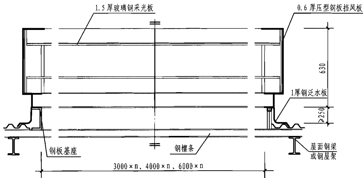
1-1 剖面图
