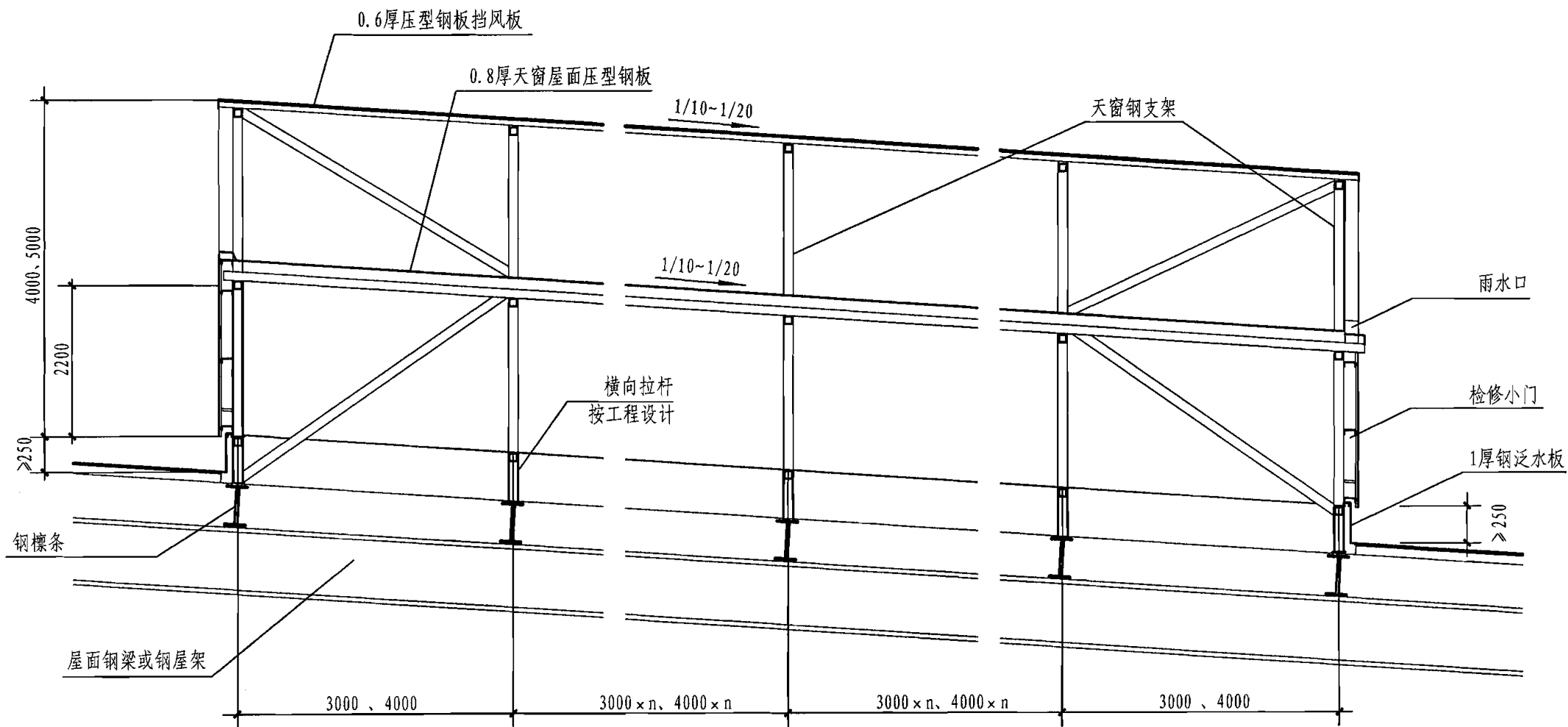
A-A剖面图
