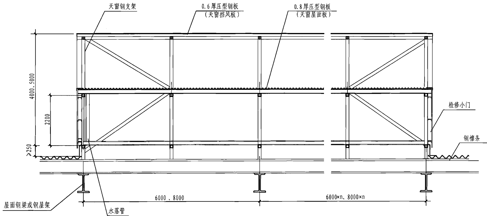
A-A剖面图
