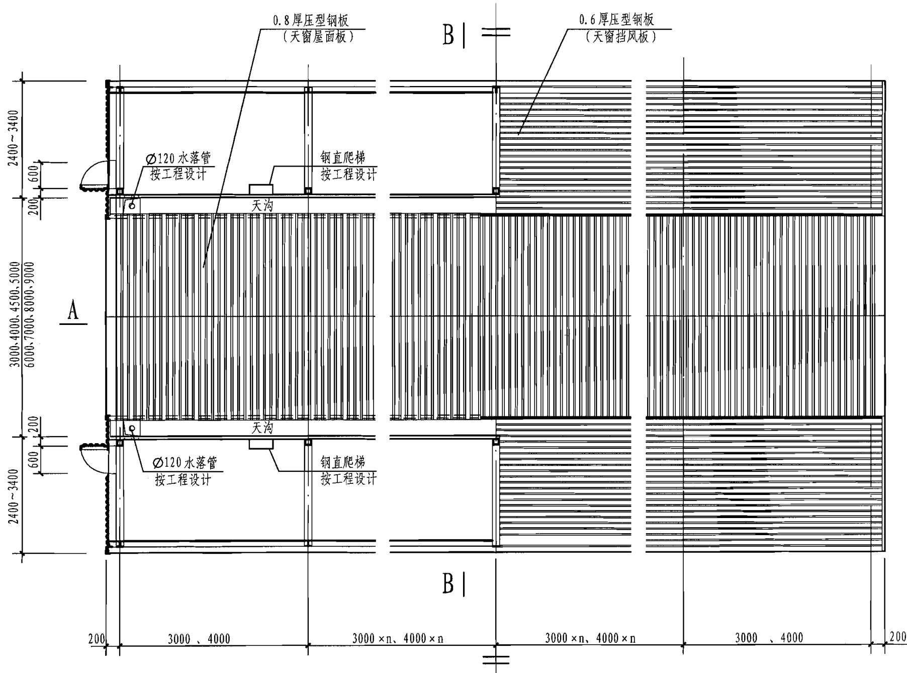
天窗平面图
