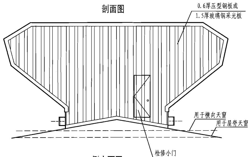
侧立面图
