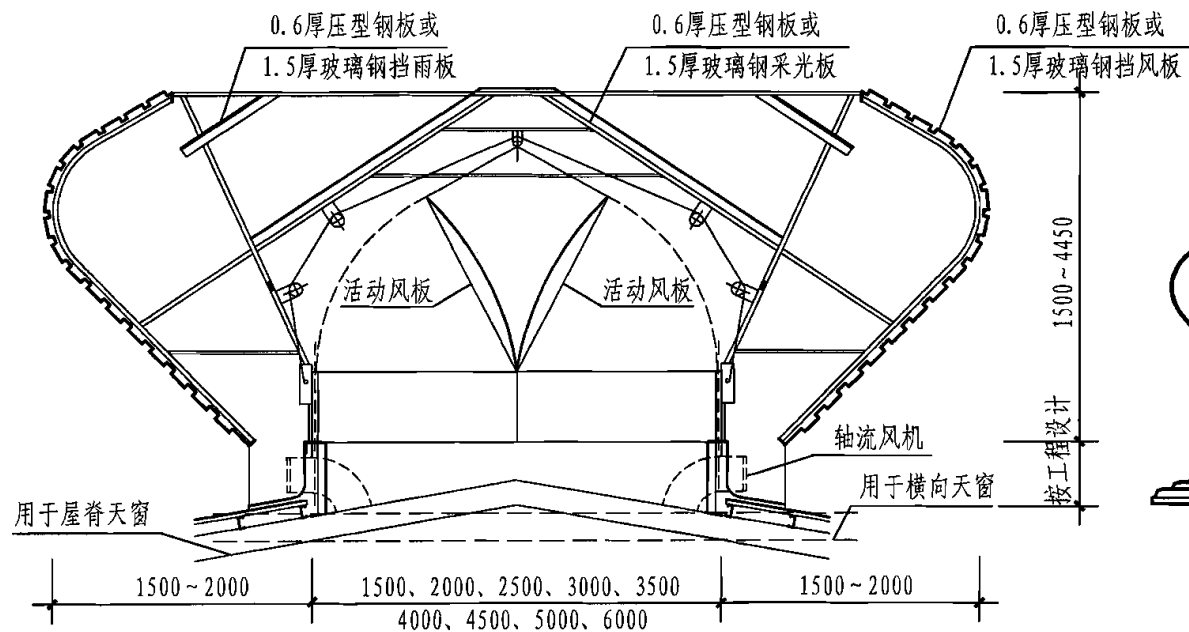
剖面图
