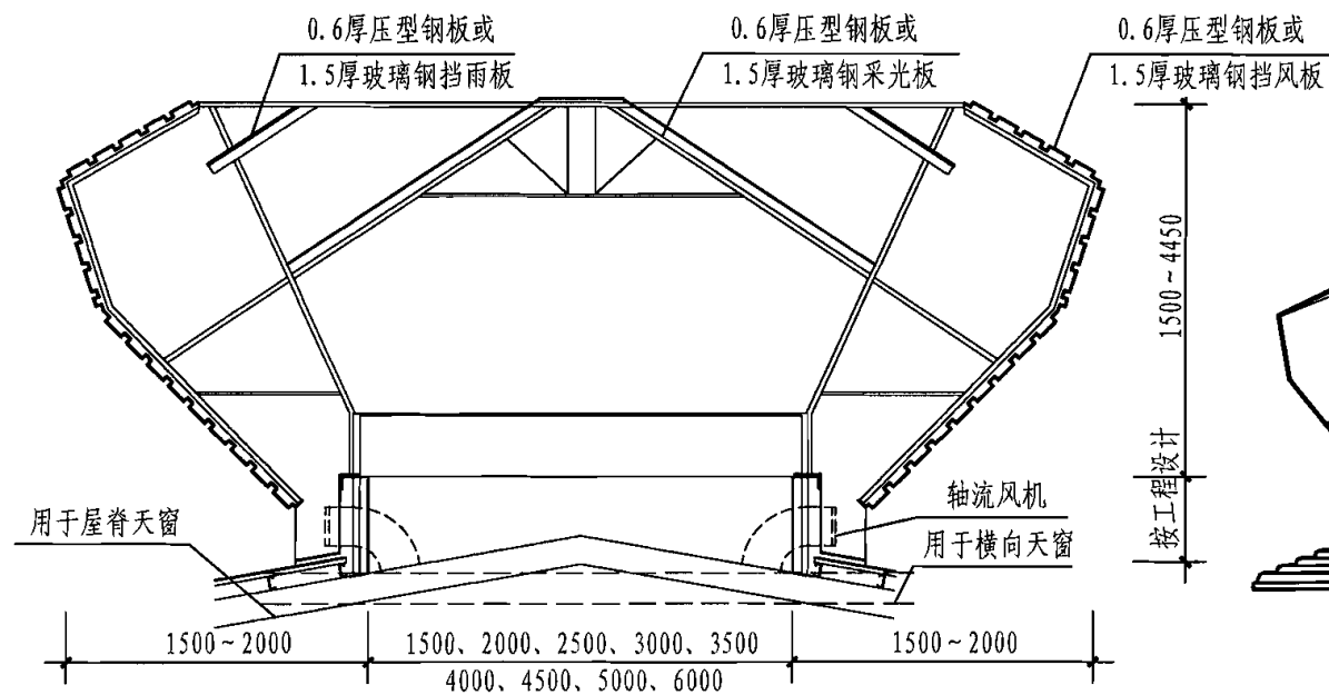
剖面图
