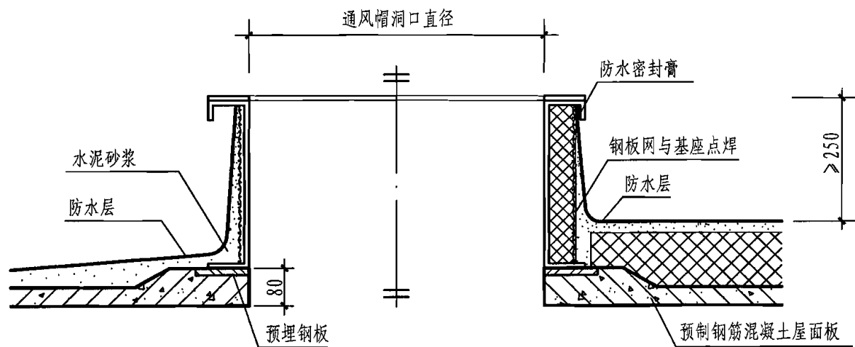
2-2剖面图
