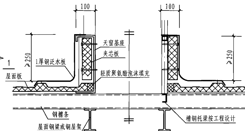
3-3 剖面图
