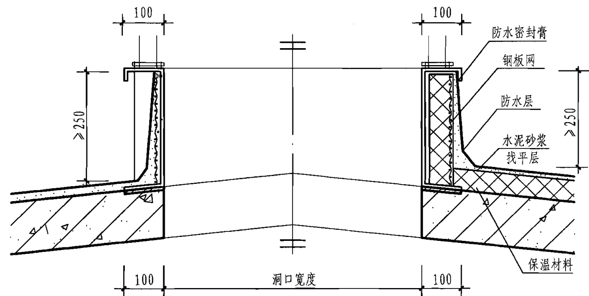
1-1 剖面图
