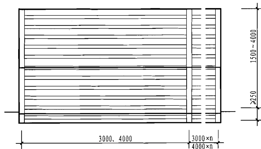
立面图
