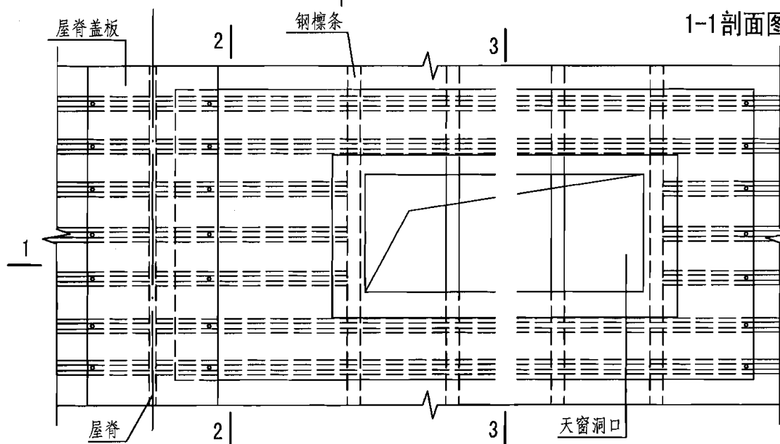
天窗基座洞口平面图
