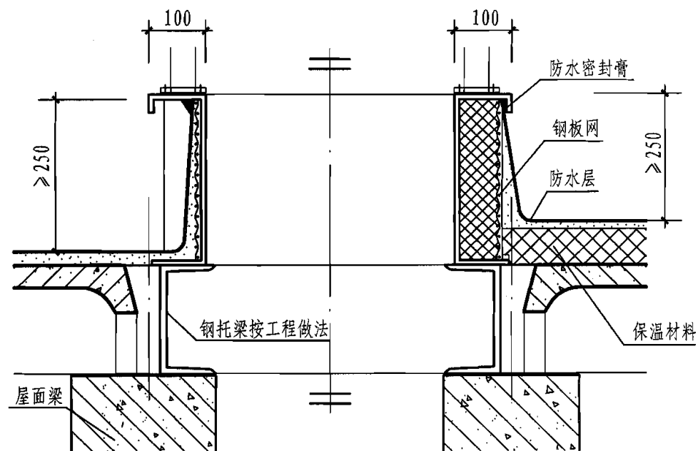
2-2 剖面图
