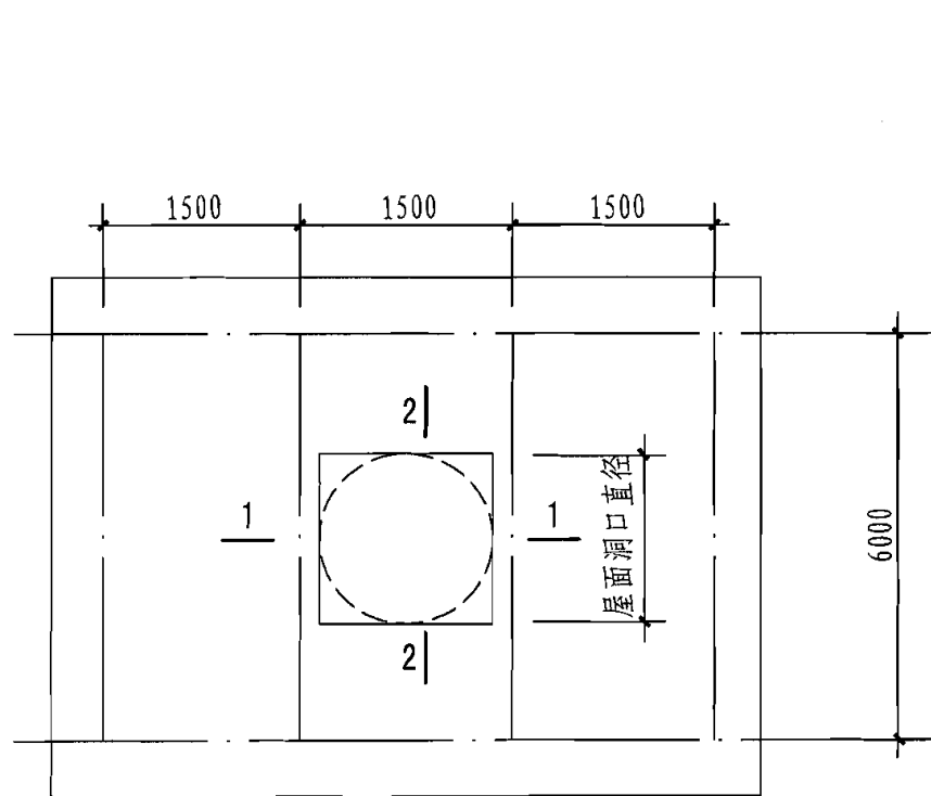
预制钢筋混凝土屋面板 通风帽安装平面示意图
