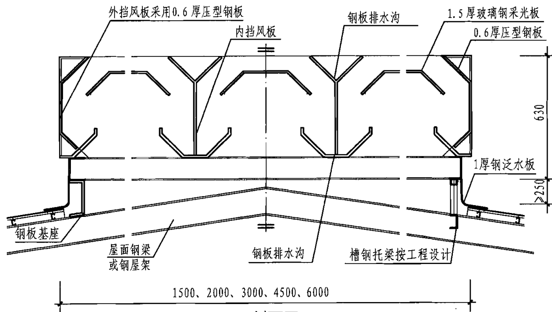
2-2 剖面图
