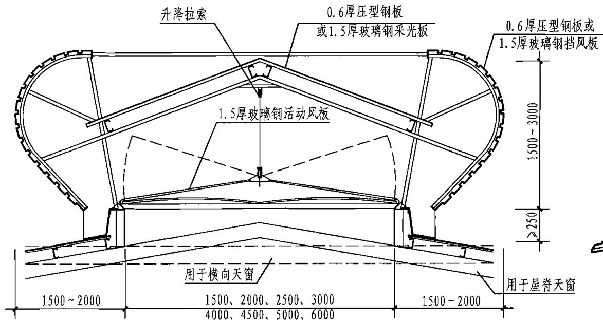
剖面图
