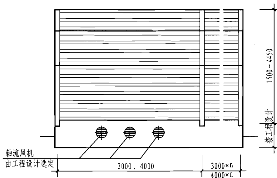
立面图
