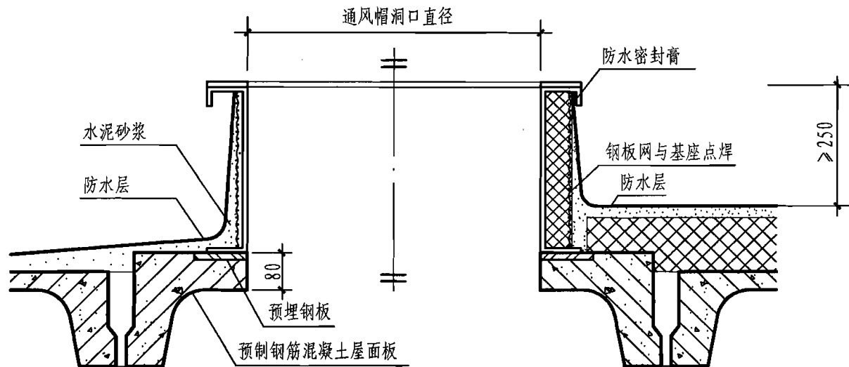
1-1剖面图
