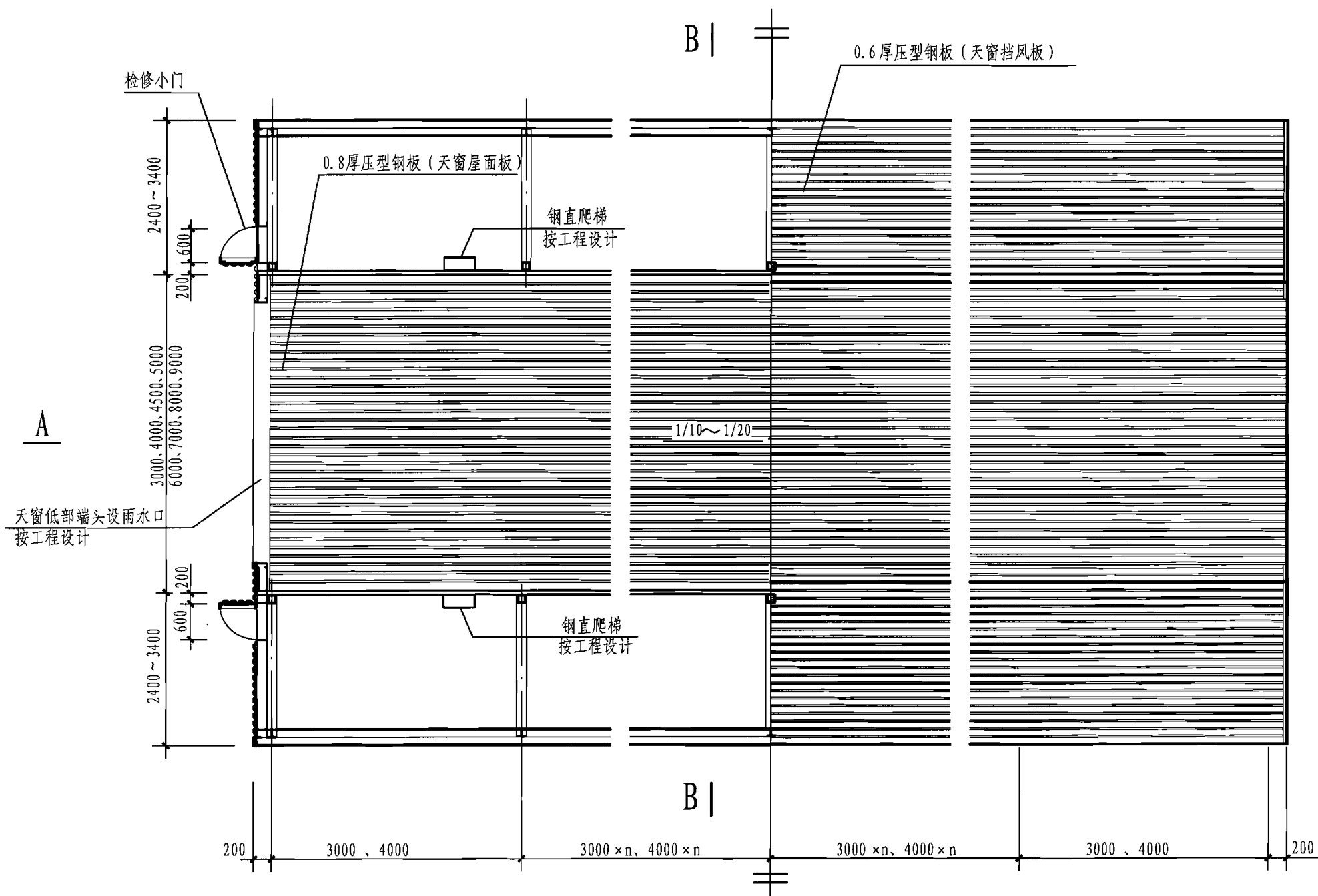
平面图
