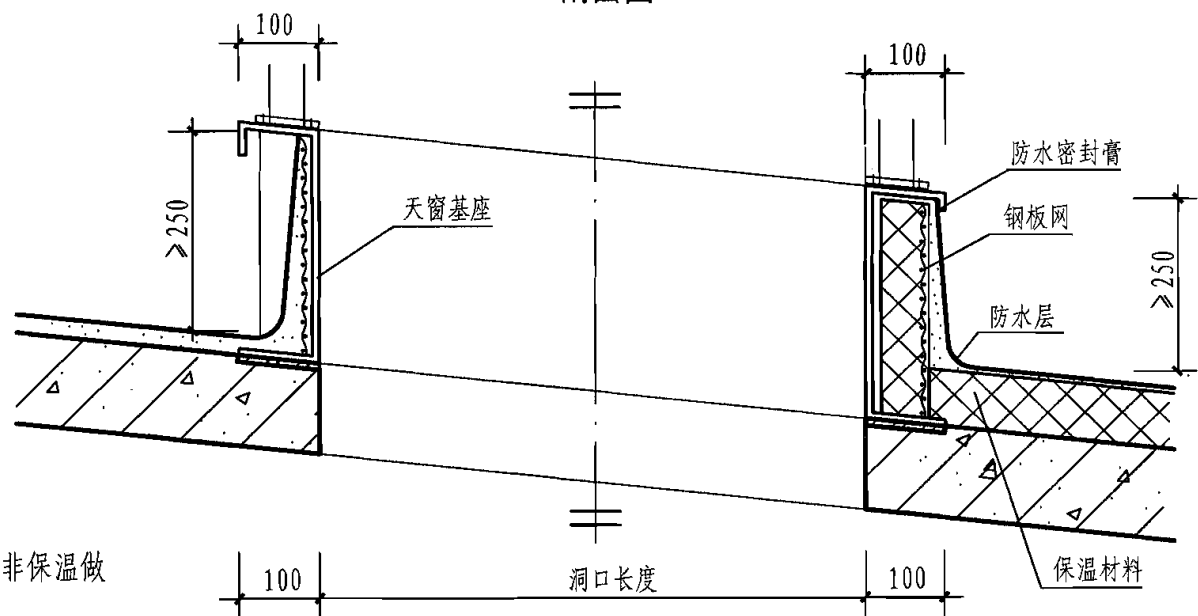
2-2 剖面图
