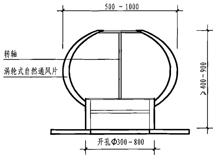
剖面图
