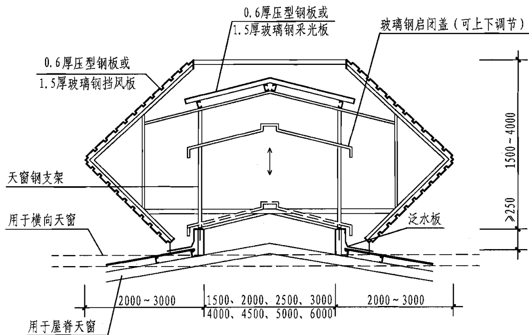
剖面图
