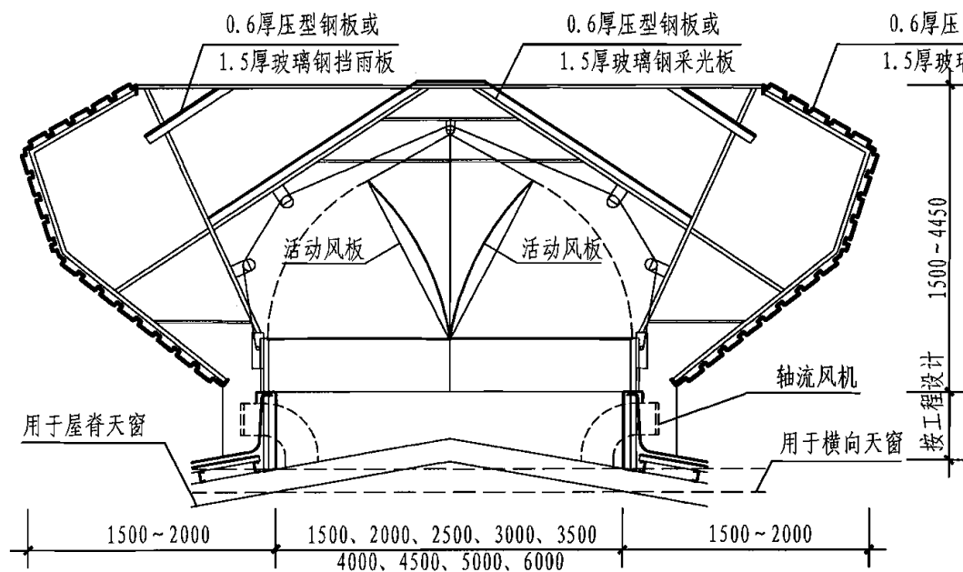
剖面图
