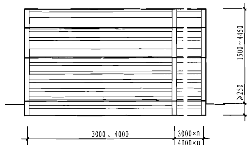
立面图
