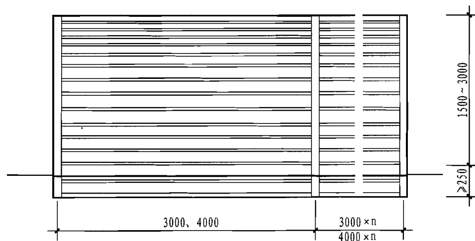
立面图
