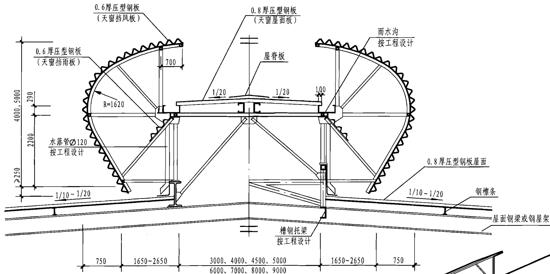
B-B 剖面图
