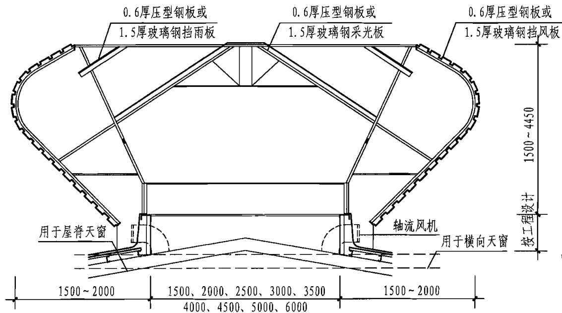
剖面图
