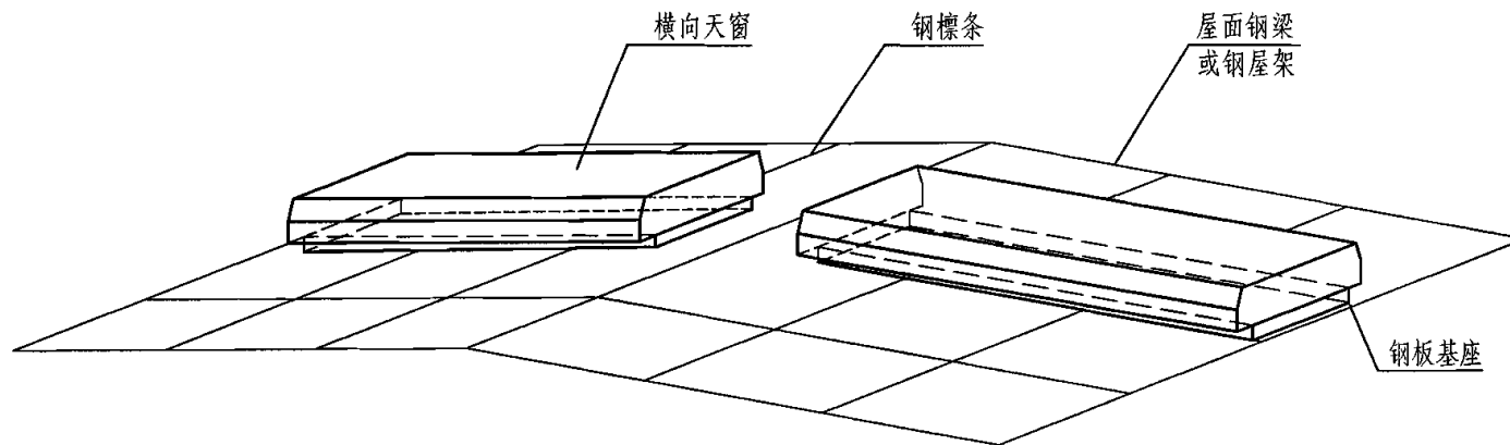
横向天窗示意图
