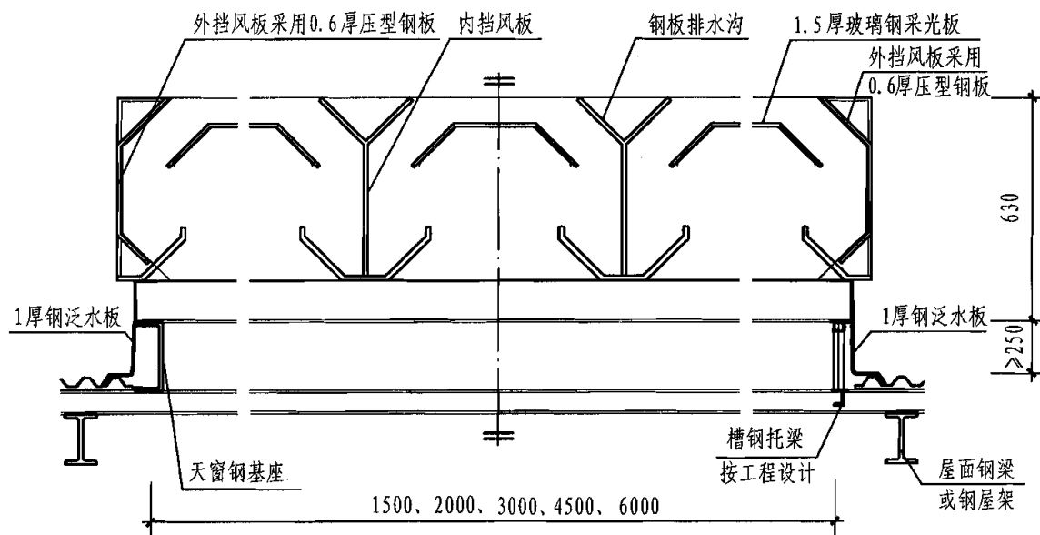
2-2 剖面图
