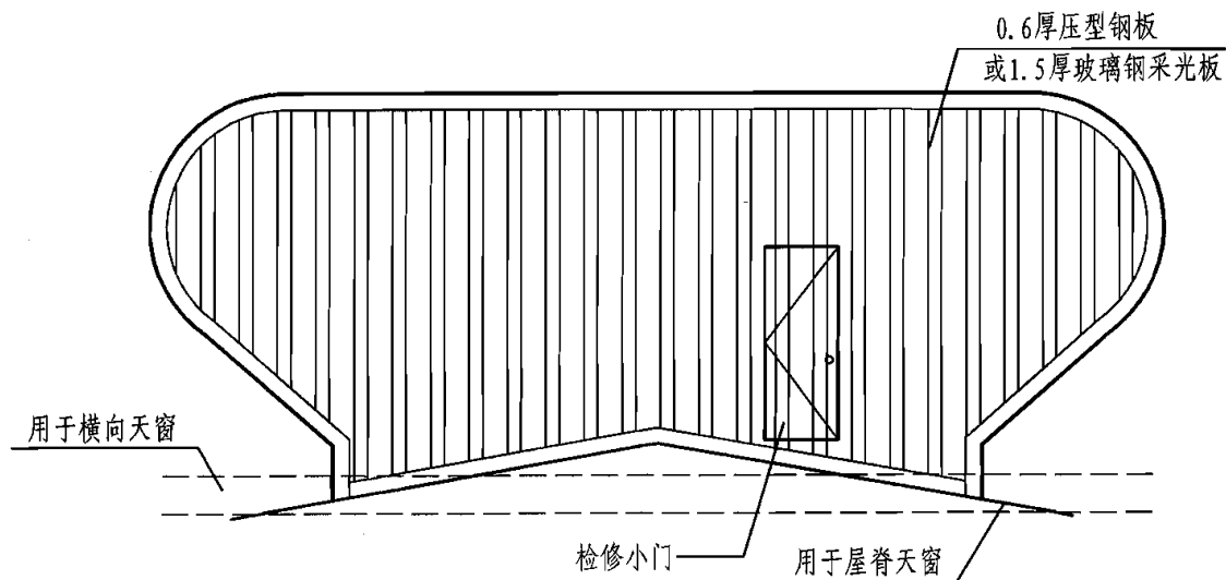
侧立面图
