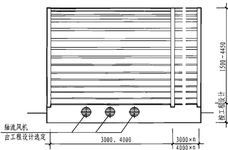
立面图
