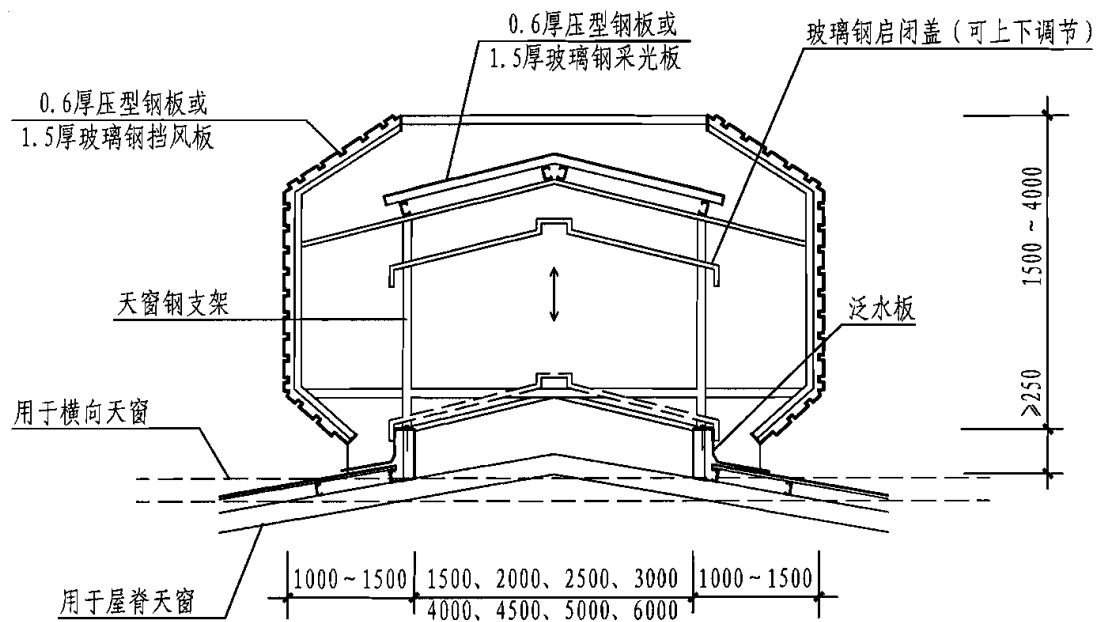
剖面图
