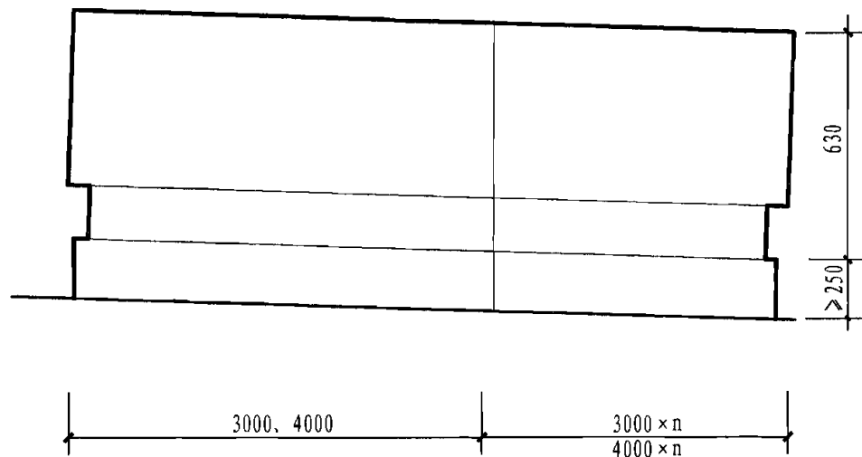
立面图
