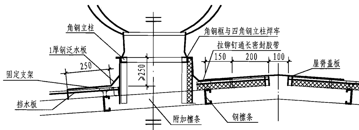
1-1 剖面图
