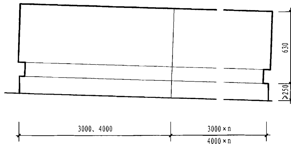
立面图
