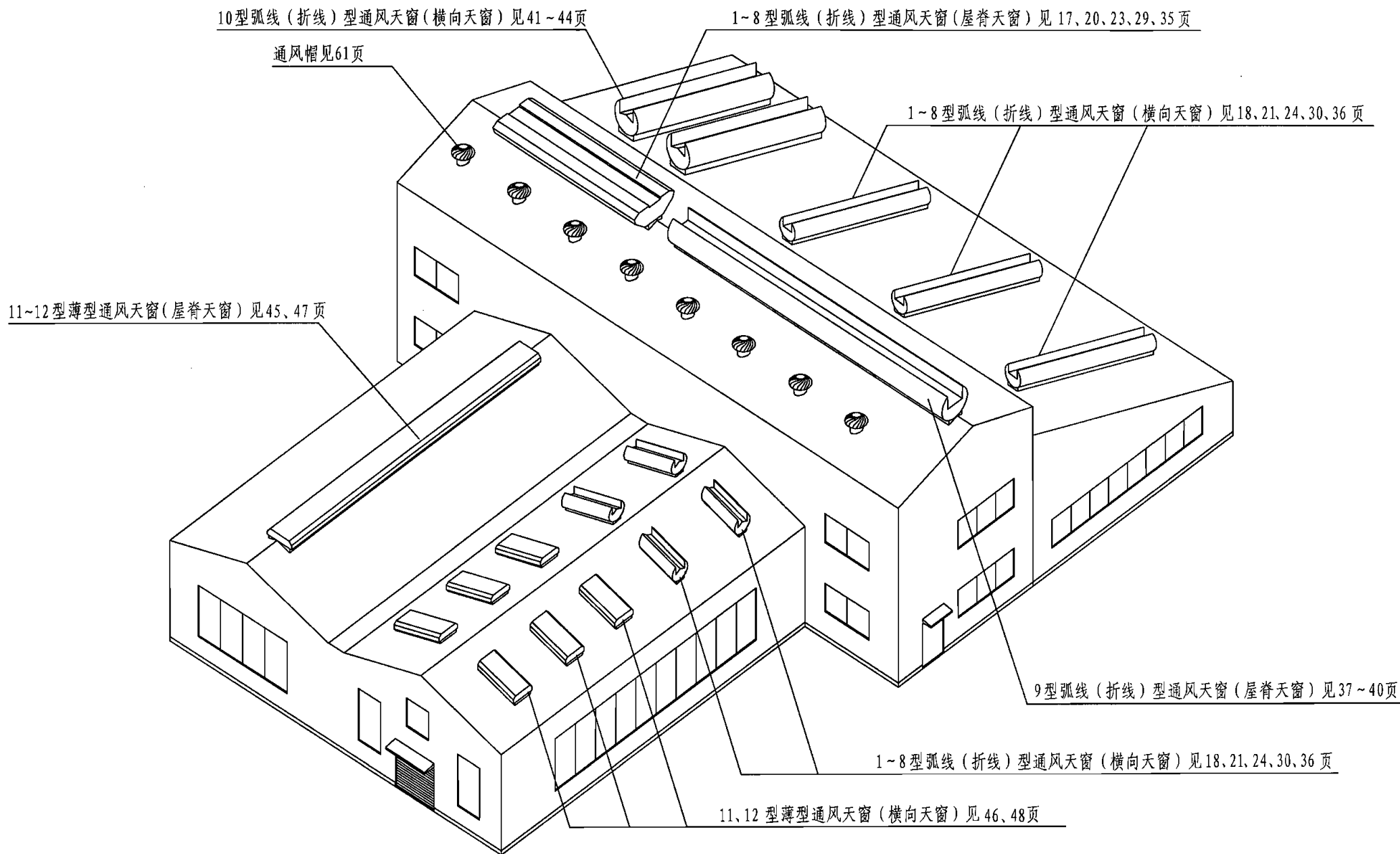
通风天窗选用示意图
