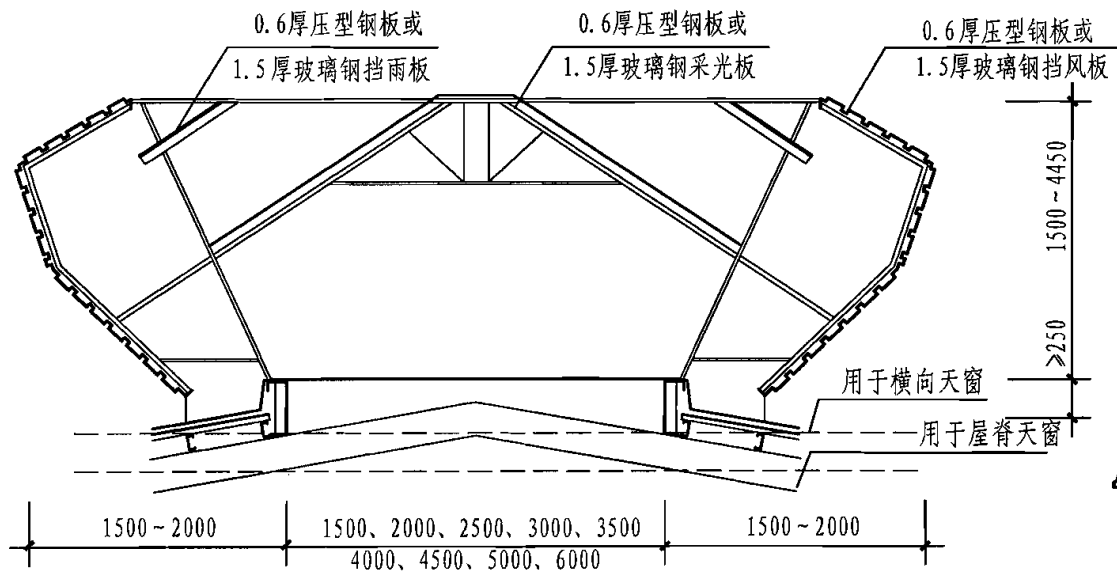
剖面图
