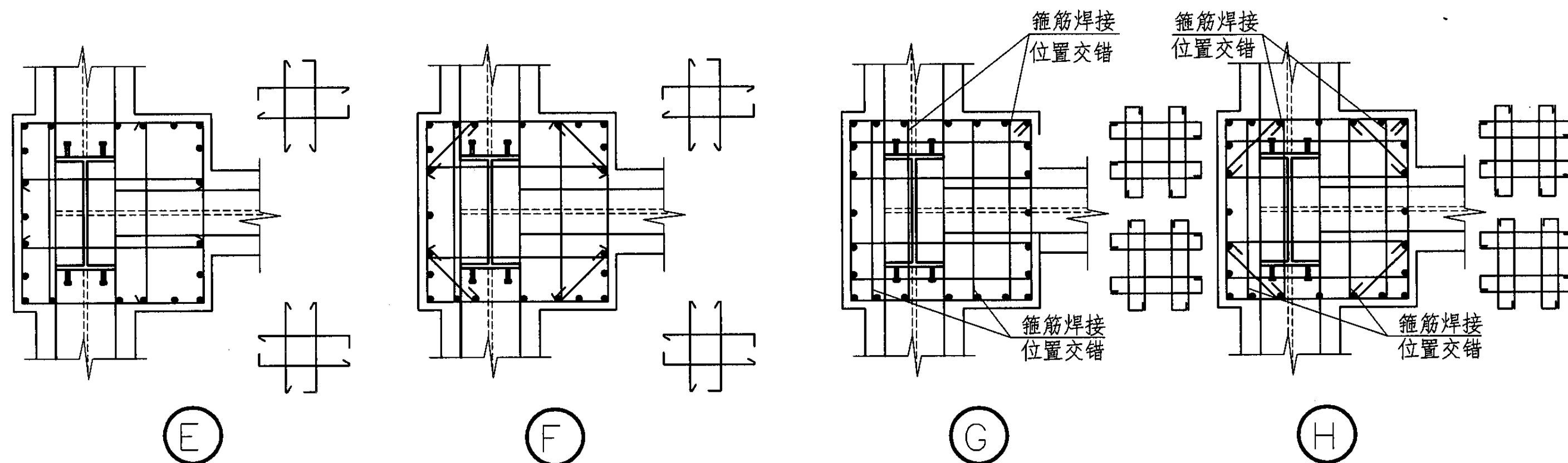
型钢混凝土边柱节点区箍筋连接示意图
