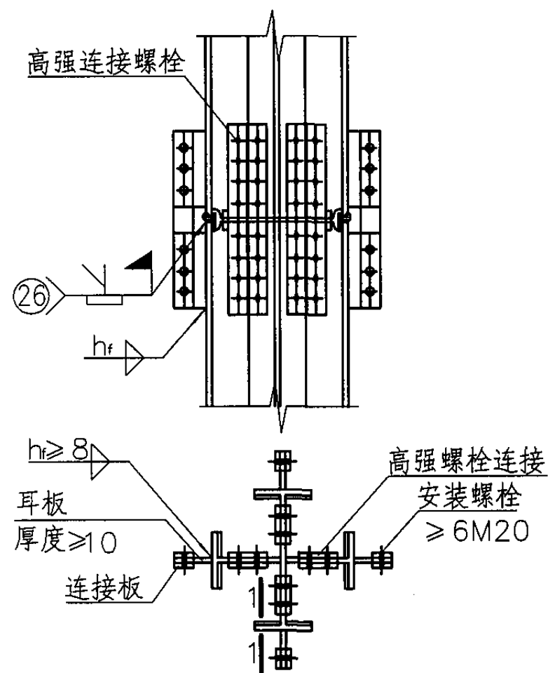
十字形截面柱拼接节点1
