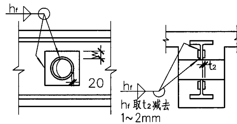
腹板开圆孔的钢板补强构造
