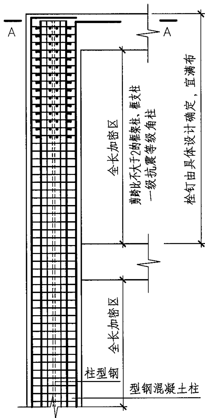
型钢混凝土角柱抗震构造
