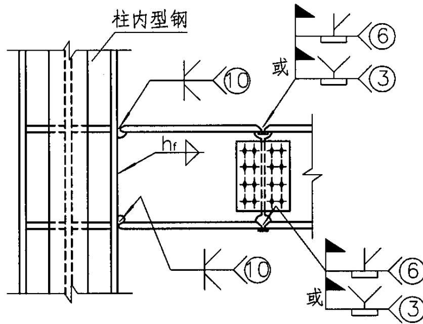
梁柱节点构造(二)
