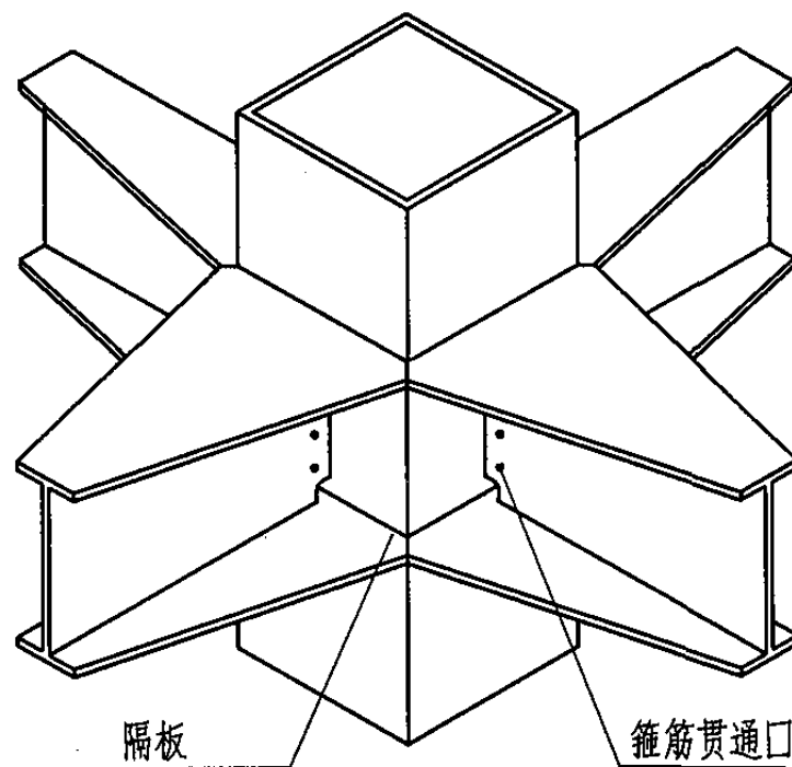
型钢梁、柱节点外隔板形式
