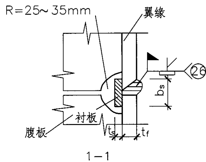
翼缘焊接, 腹板高强螺栓连接
