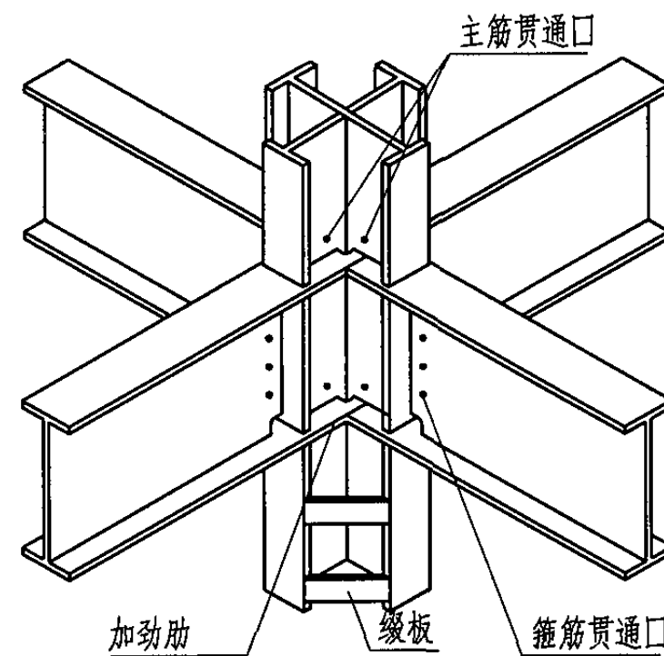
型钢梁、柱节点 梁翼缘贯通形式
