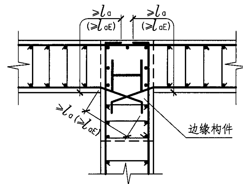
转角3
