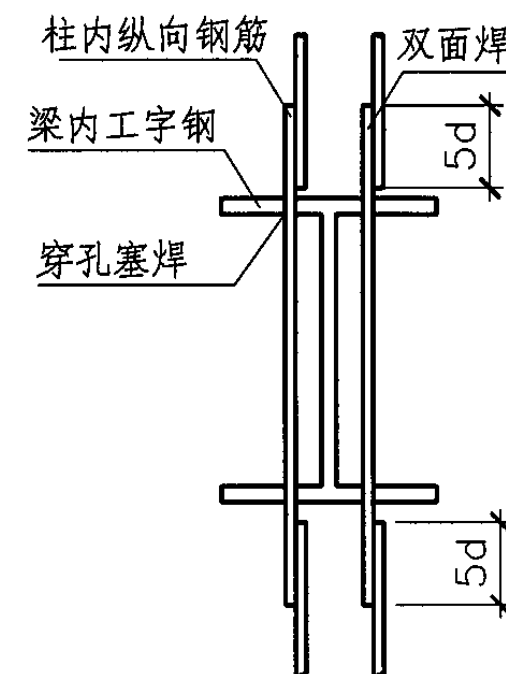
柱钢筋穿梁翼缘做法
