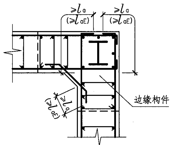
转角2
