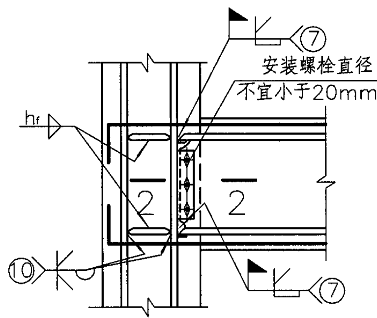
⑤ 工地焊接刚接连接(二)
