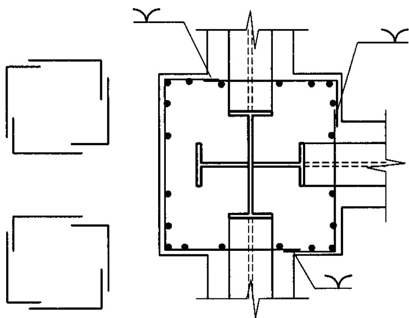
边柱1
