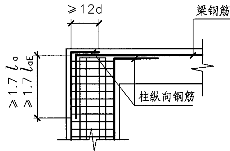
型钢混凝土柱顶层端节点锚固 2
