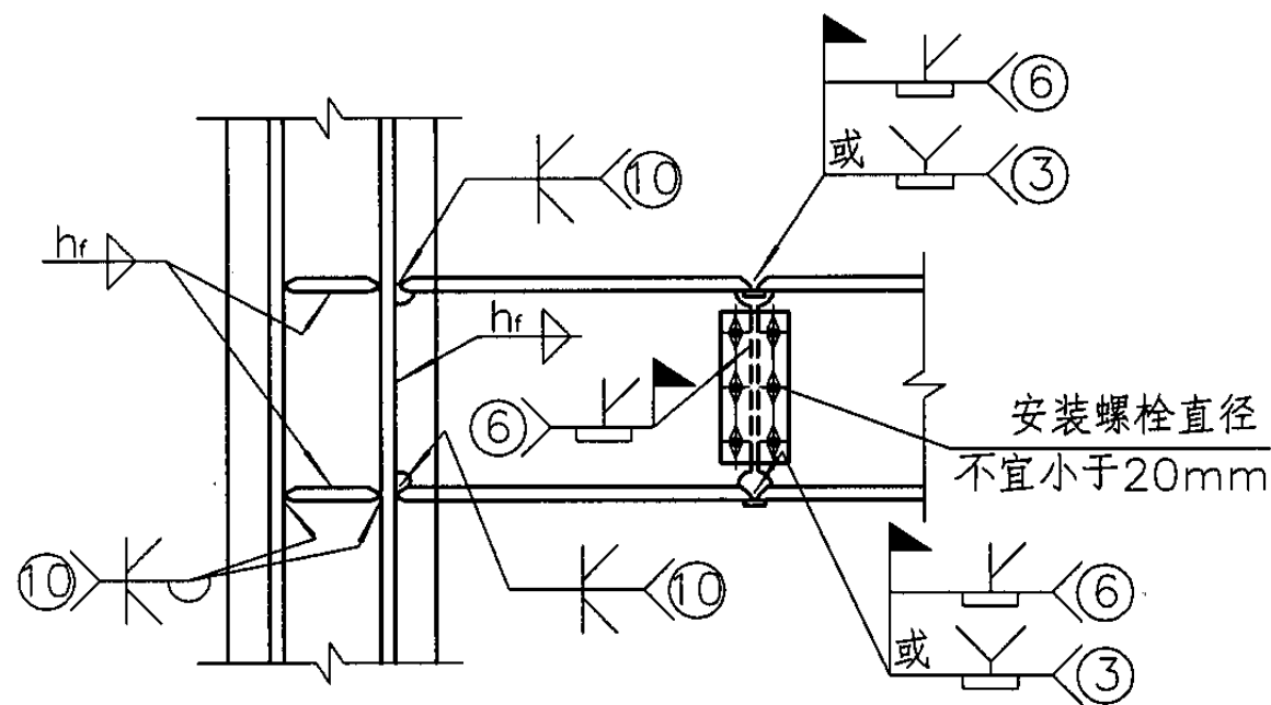
① 悬臂梁段刚接连接(一)
