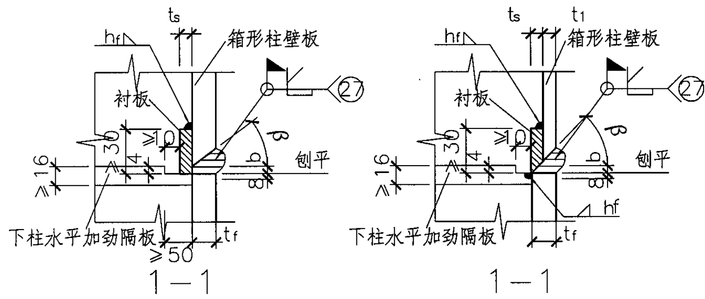
箱形柱不等厚壁板的焊接
