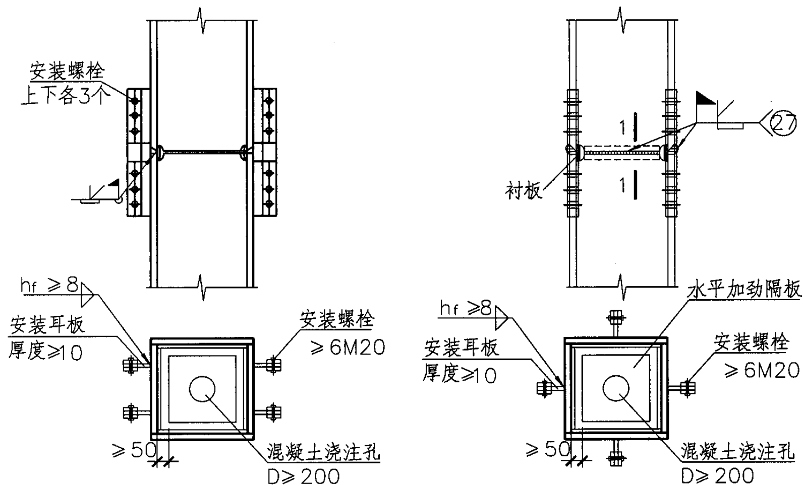
箱形截面柱拼接节点
