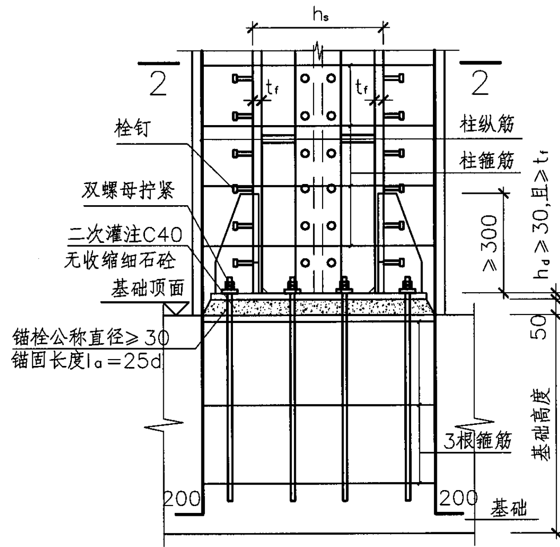
十字型型钢混凝土柱非埋入式柱脚
