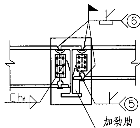
④ 两端梁不等高连接(二)
