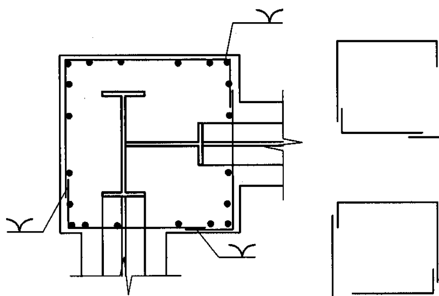
角柱2
