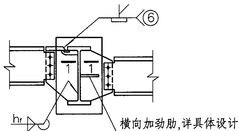
③ 两端梁不同标高的连接
