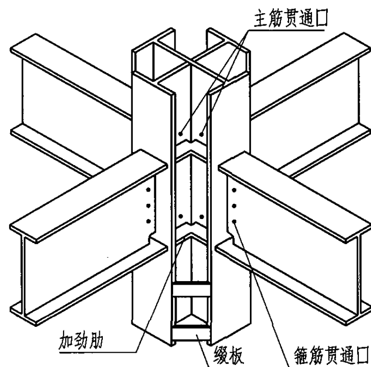
型钢梁、柱节点 水平加劲肋形式
