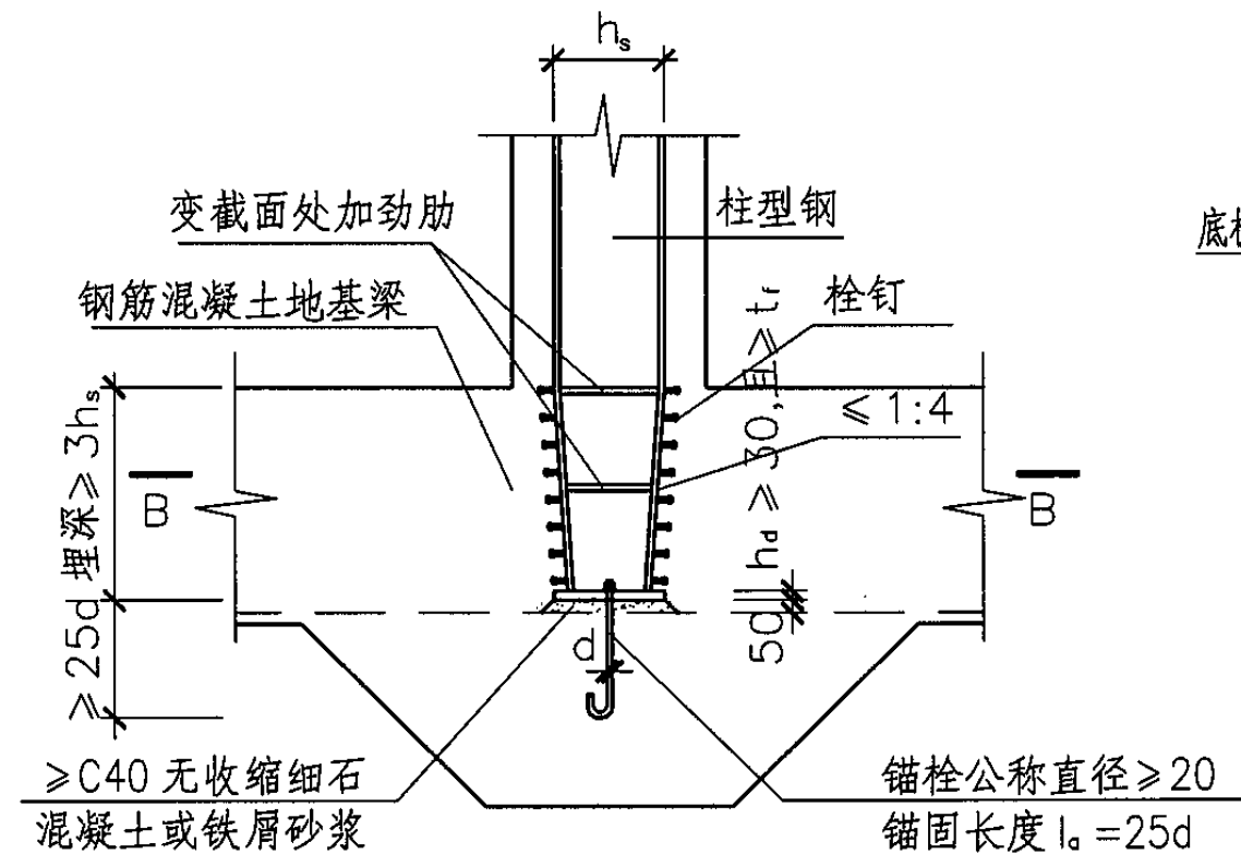
型钢混凝土柱型钢柱脚做法
