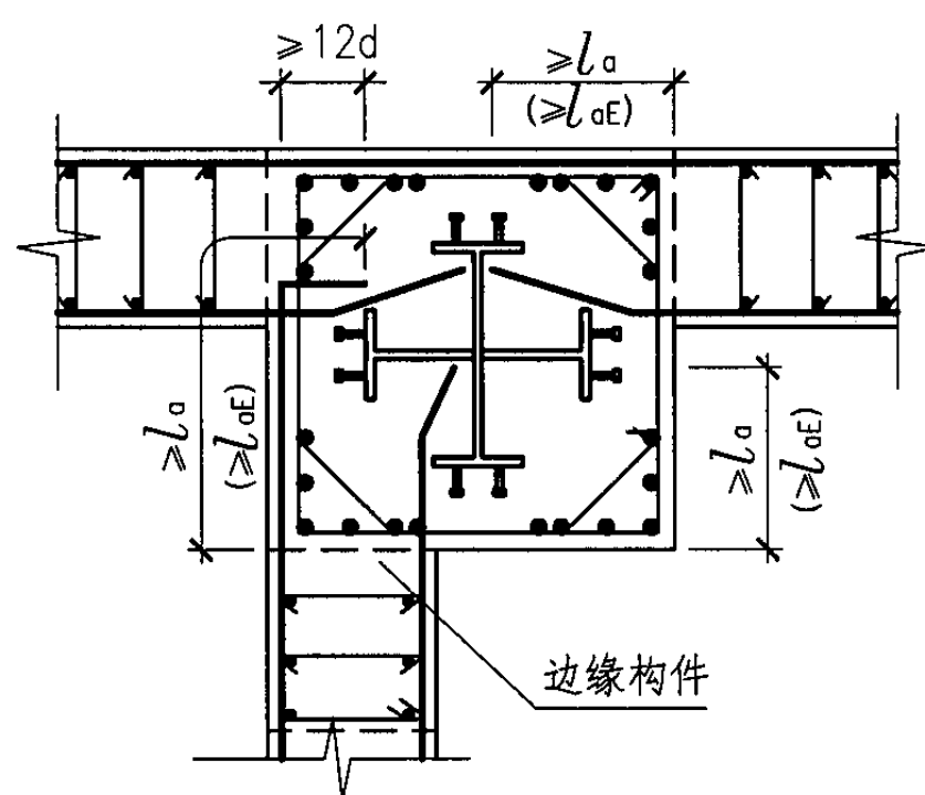
转角5
