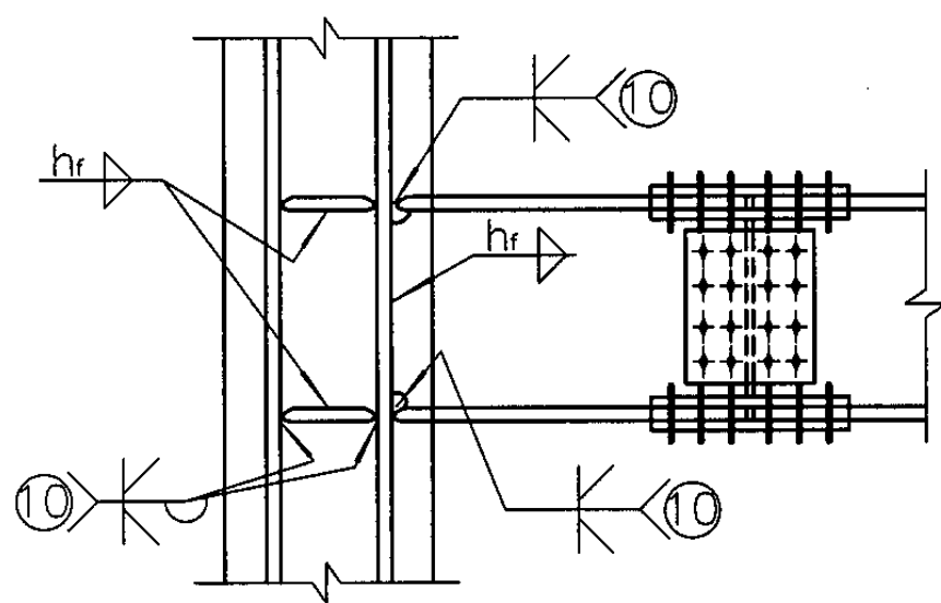
③ 悬臂梁段刚接连接(三)
