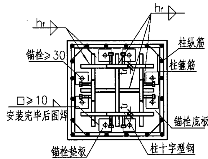
十字型型钢混凝土柱非埋入式柱脚
