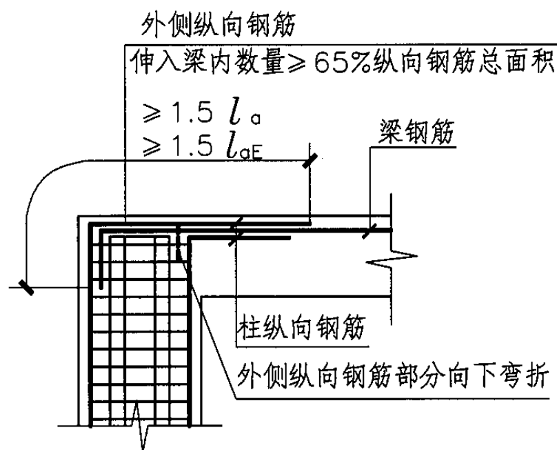
型钢混凝土柱顶层端节点锚固 1
