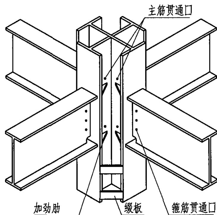
型钢梁、柱节点 水平三角加劲肋形式
