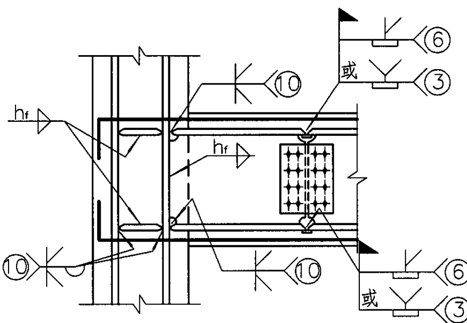
② 悬臂梁段刚接连接(二)
