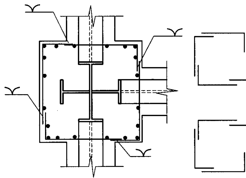
边柱2
