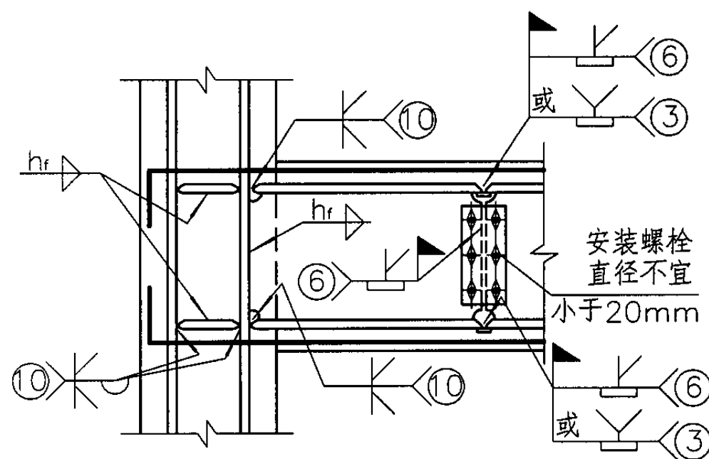
① 悬臂梁段刚接连接(一)
