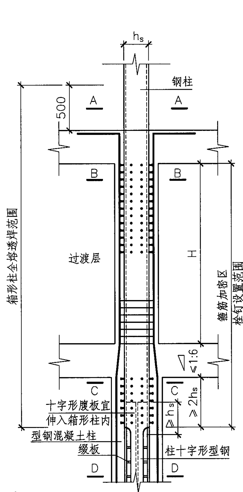
2 型钢混凝土柱与钢柱的过渡层构造
