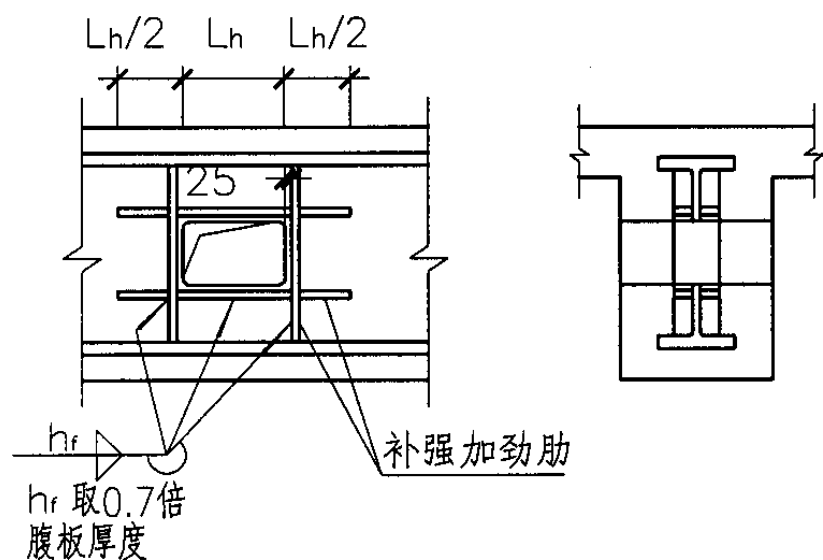
腹板开矩形孔的加劲肋补强构造
