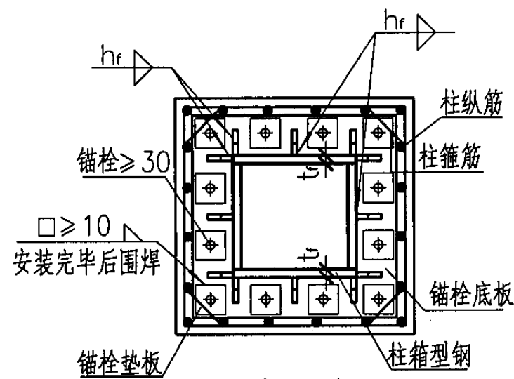
1-1 用于锚栓拉力大的情况 栓钉未表示
