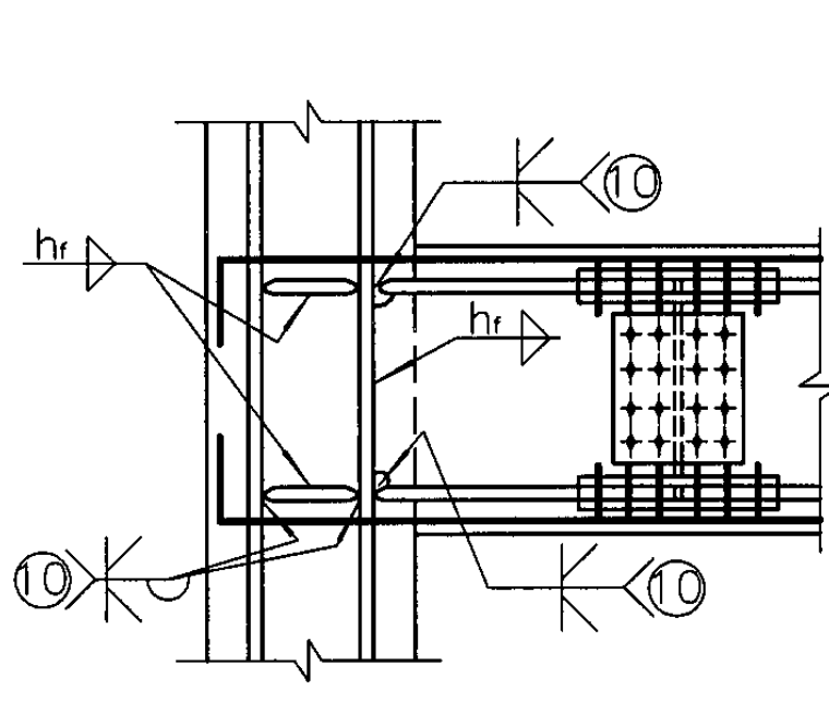
③ 悬臂梁段刚接连接(三)
