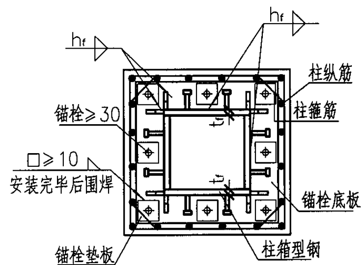
1-1 用于锚栓拉力小的情况
