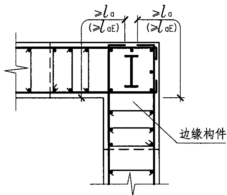
转角1
