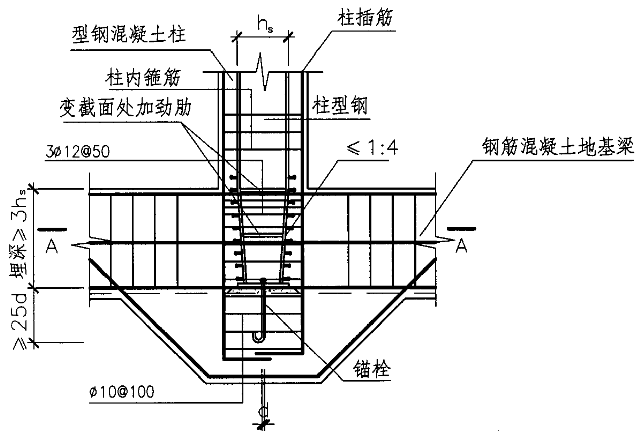
型钢混凝土柱埋入式柱脚(二)
