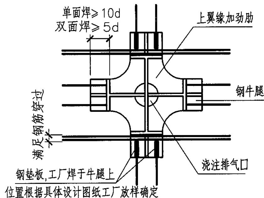
上翼缘加劲肋示意图
