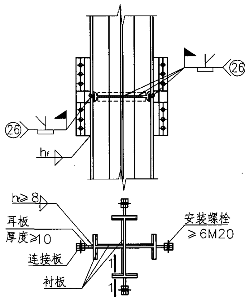
十字形截面柱拼接节点2
