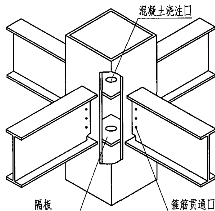
型钢梁、柱节点内隔板形式
